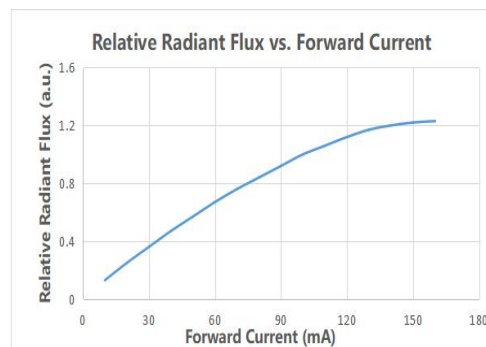
2) 正向电流与相对辐射通量特性曲线
