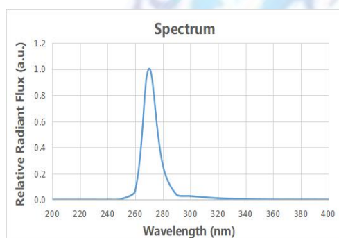
5) 光谱分布特性曲线
