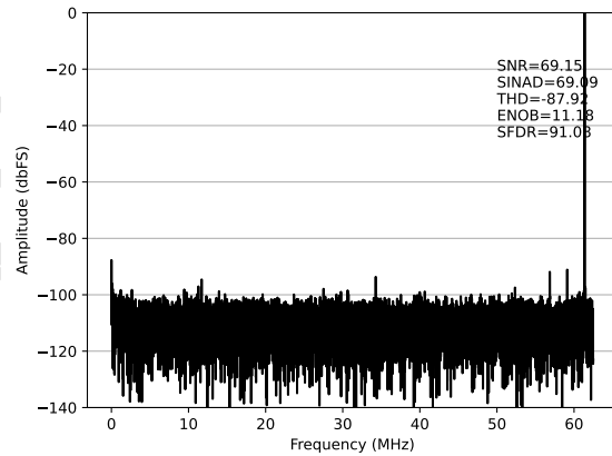
(d) 输入信号频率 = 61MHz
