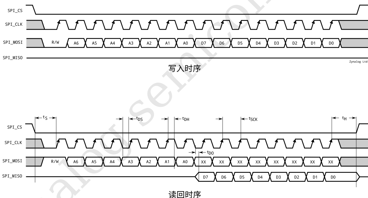
图 14: SPI 时序图
