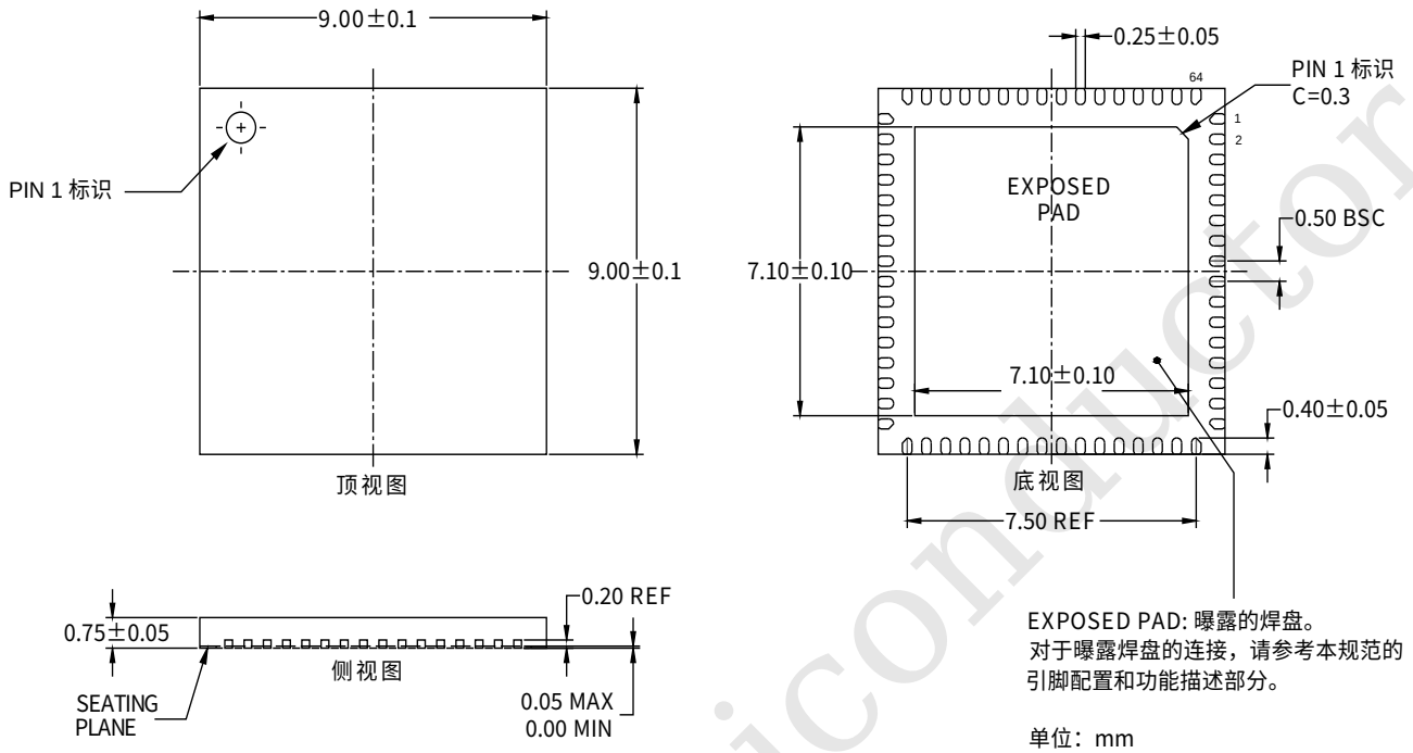
图 15: 封装信息
