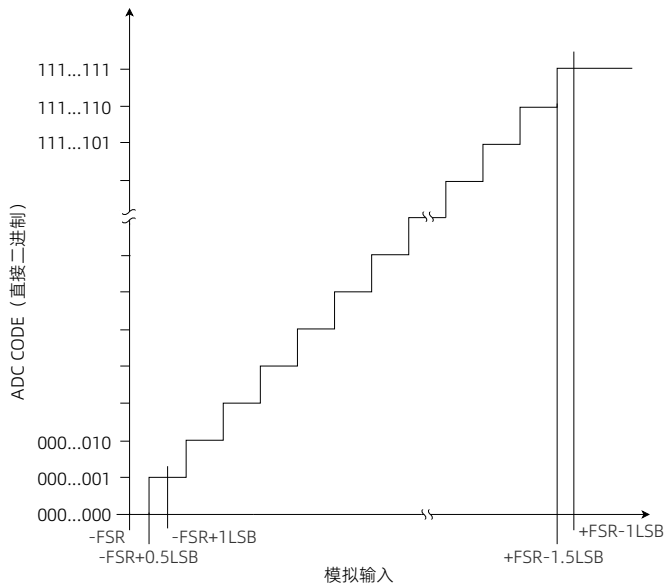
图 17 传递特性
