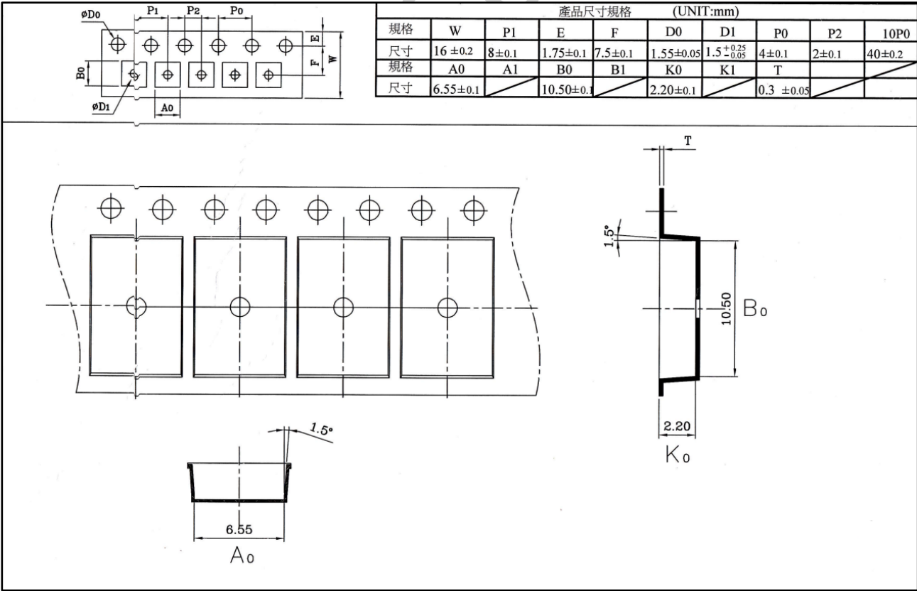
图 18. CMT804X NB SOIC-16 编带信息
