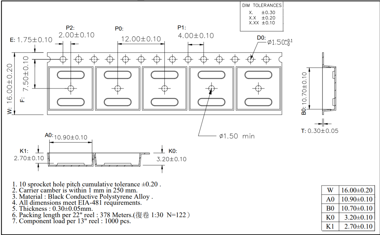
图 16. CMT804X WB SOIC-16 编带信息
