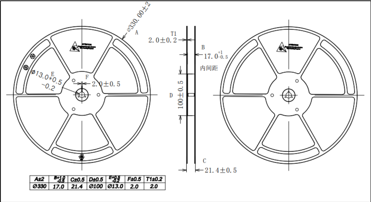
图 17. CMT804X NB SOIC-16 卷带信息
