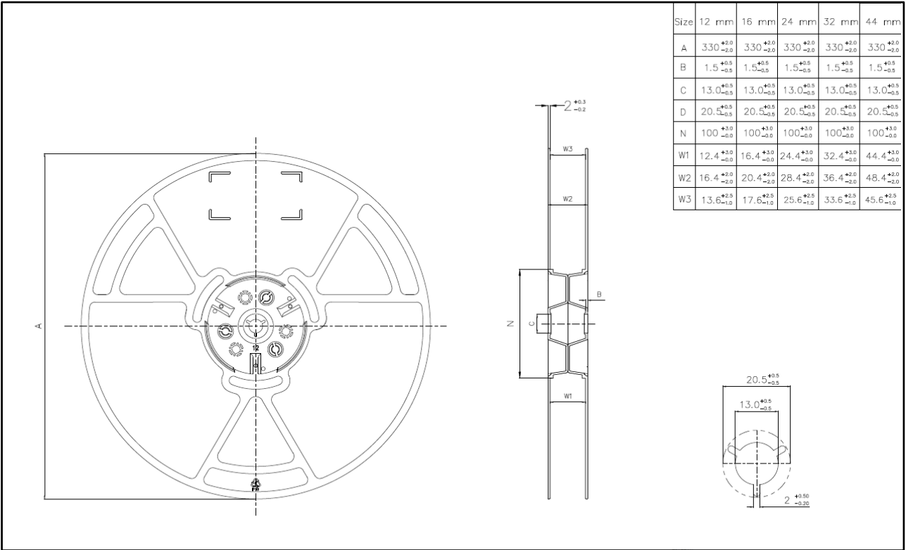
图 15. CMT804X WB SOIC-16 卷带信息
