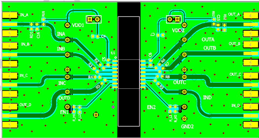
图 5. 推荐 PCB 布局
