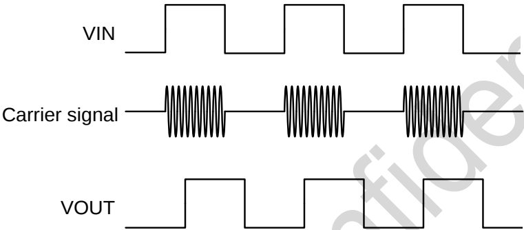
图 10.OOK 调制机制
