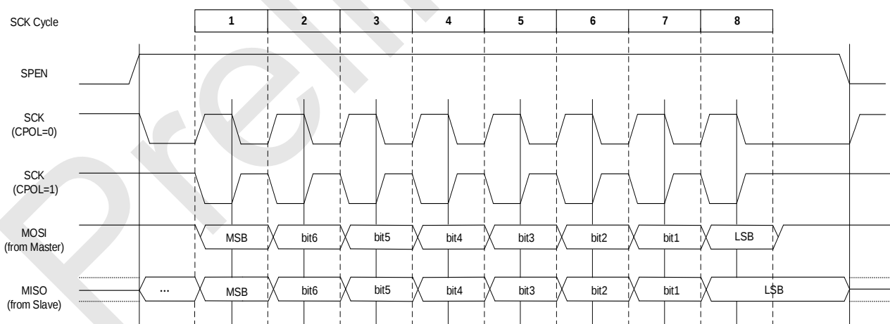
CPHA = 1 数据传输图
