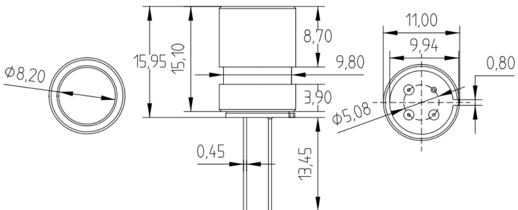
SY-TP-36BPDG-C封装尺寸
