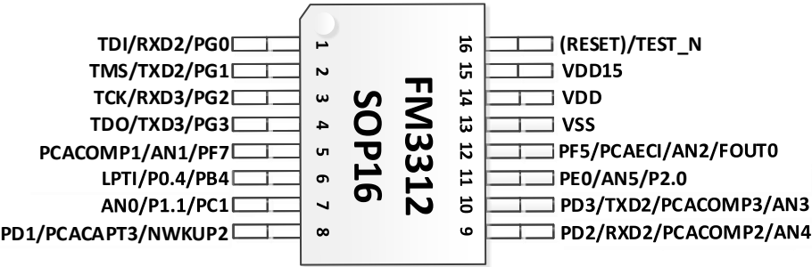
图 1-4 FM3312 封装图
