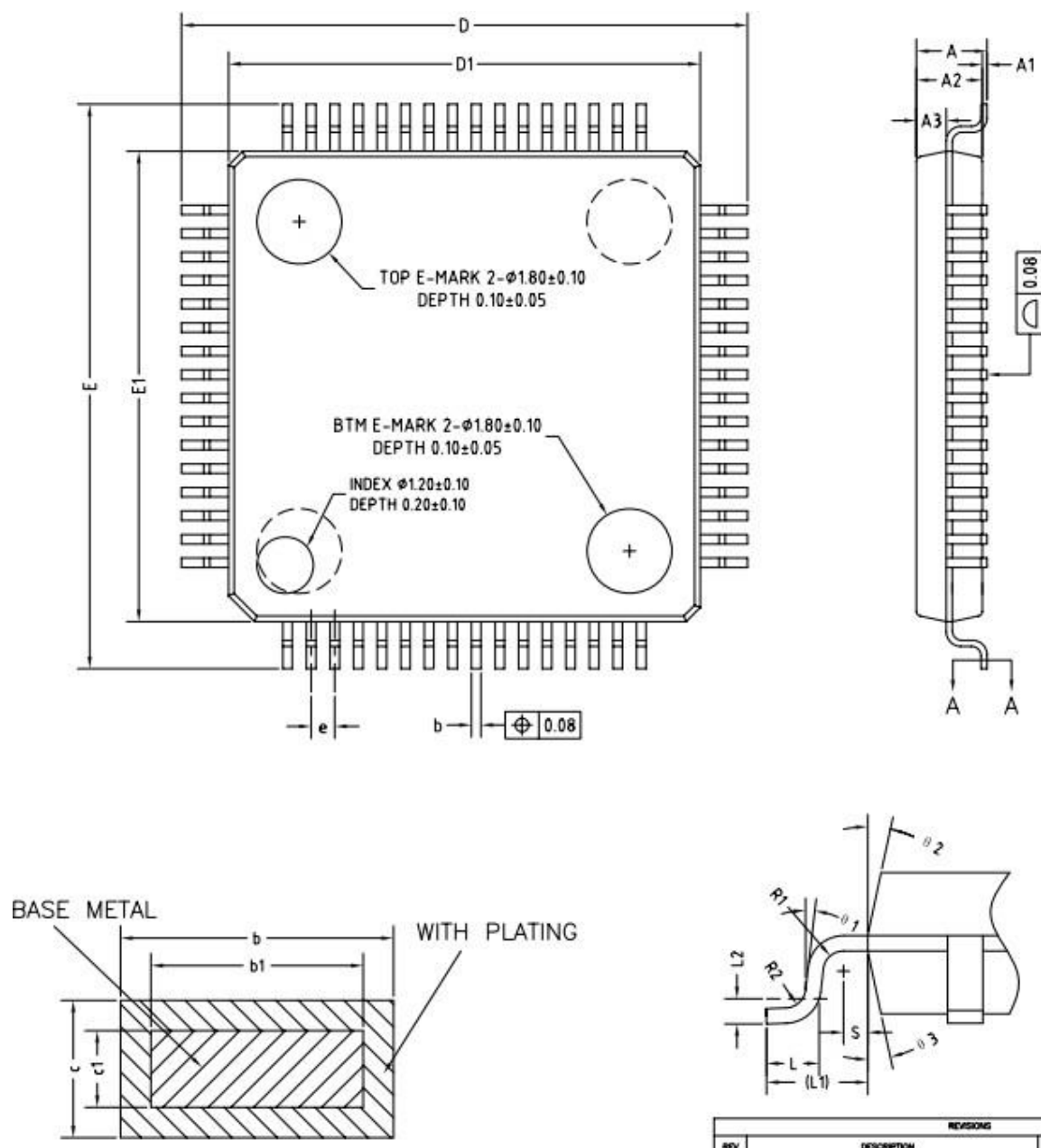
图 1-5 LQFP64 封装尺寸图
