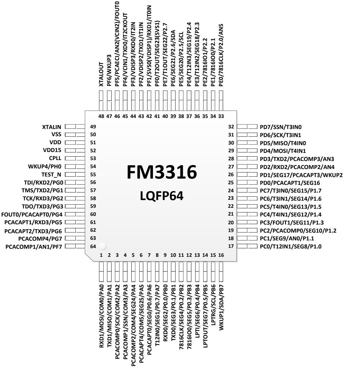
图 1-2FM3316 封装图
