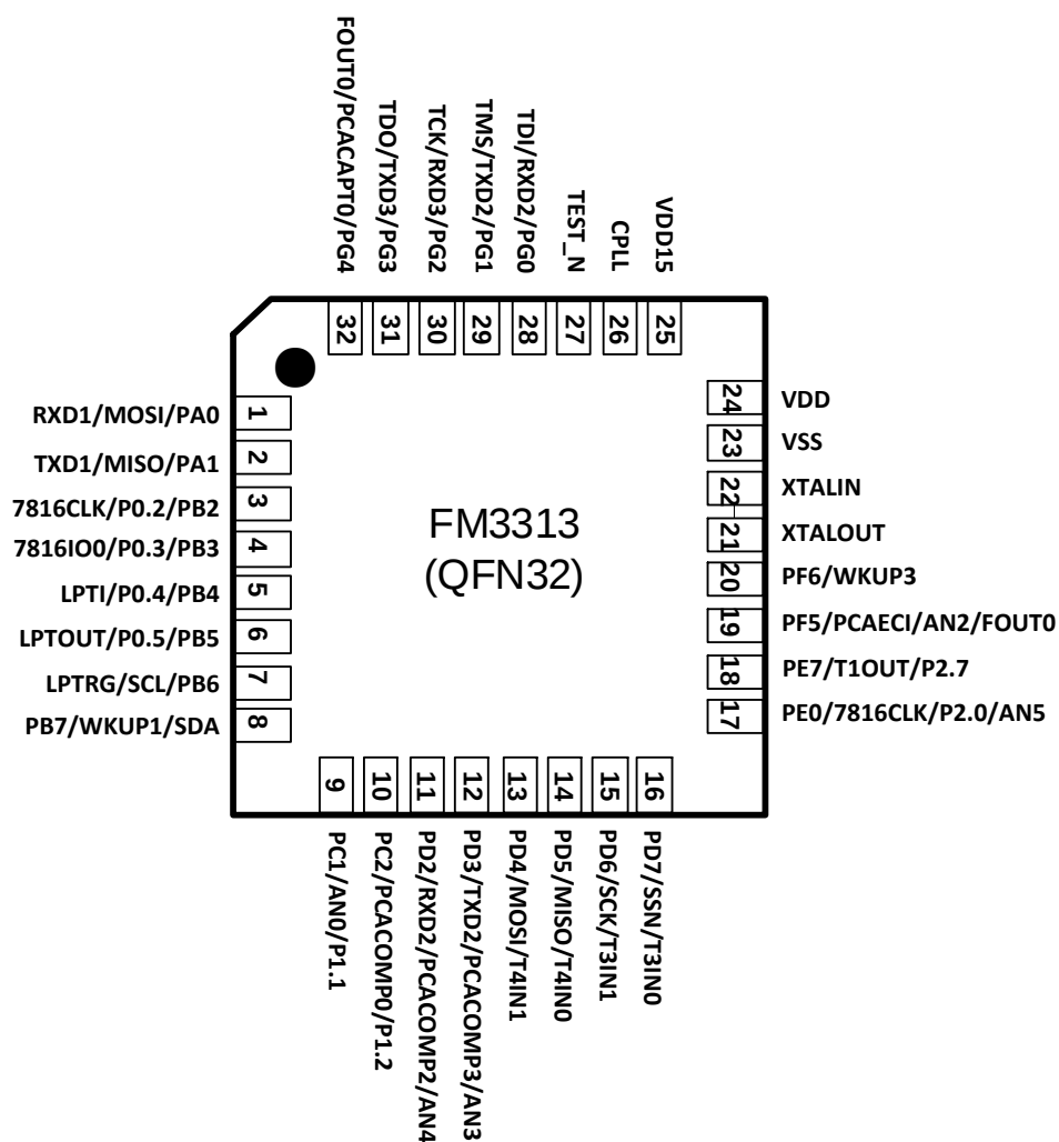
图 1-3FM3313 封装图
