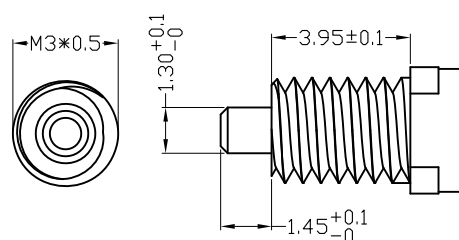
轴心部尺寸详图 2:1
