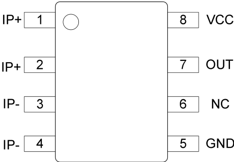
SOP8 封装
