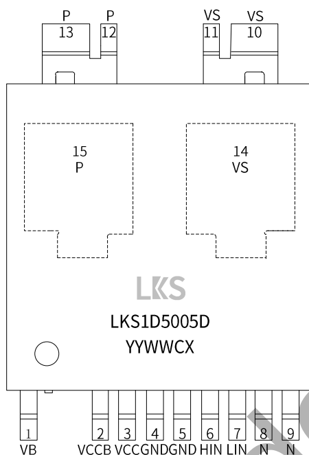
图 2. LKS1D5005DC 管脚封装图
