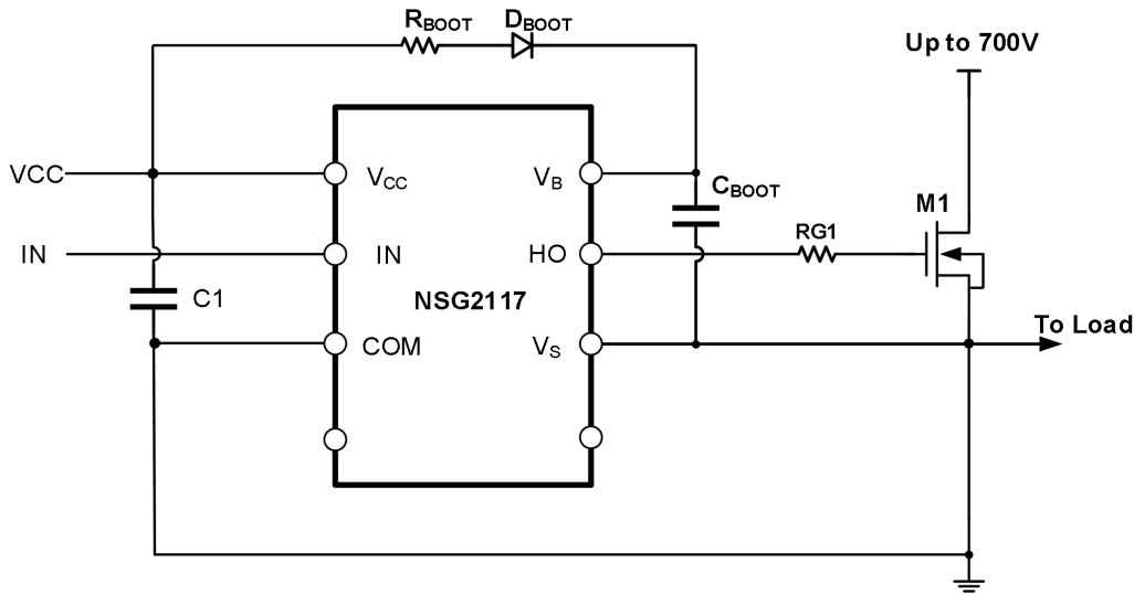
图 10-2 NSG2117 典型应用电路图
