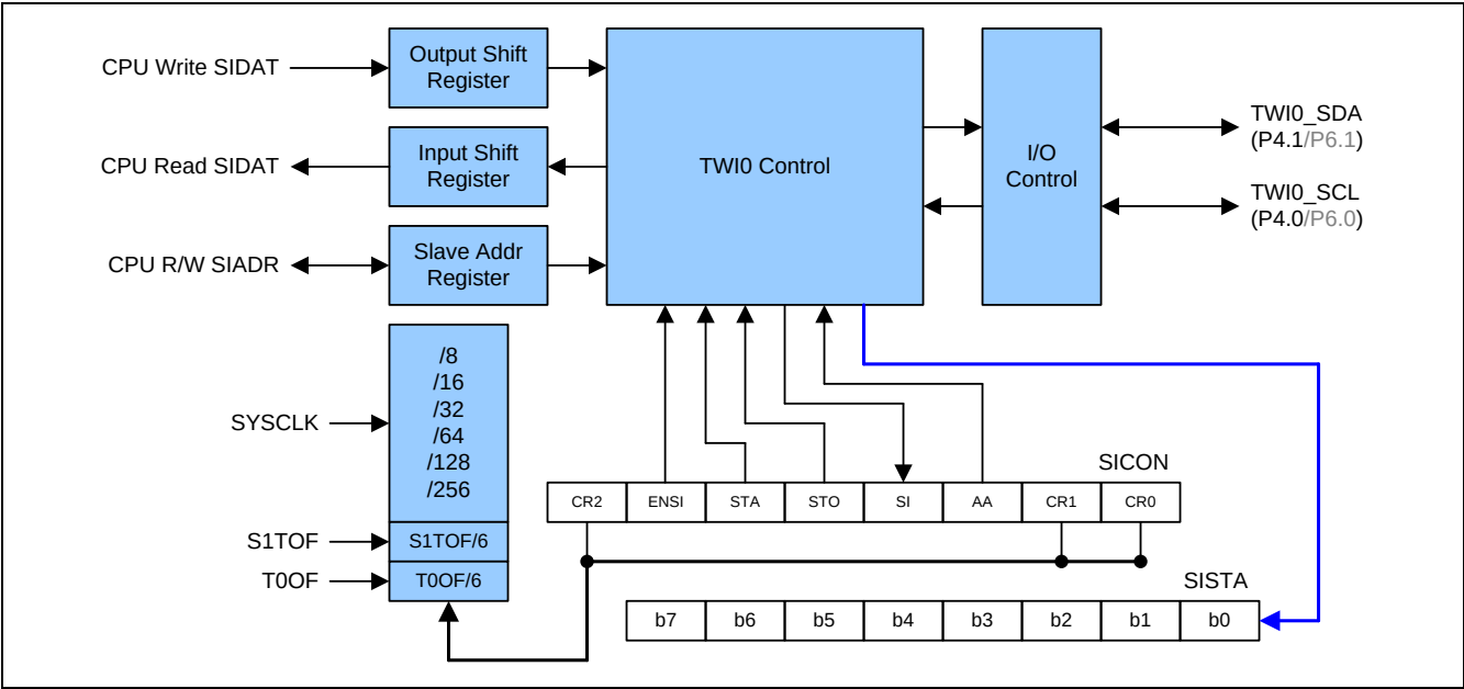
图 21-2. TWI0 功能框图
