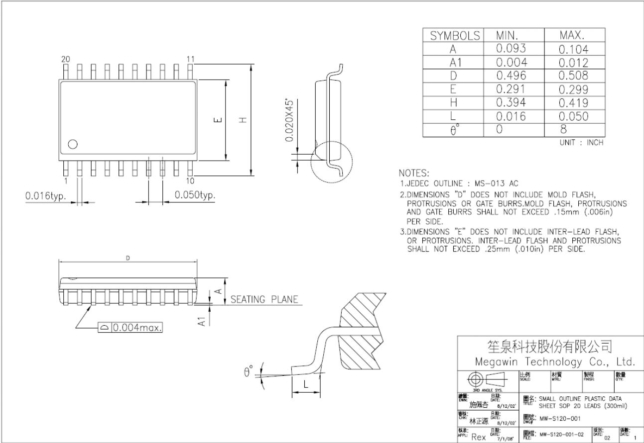
图 33-3. SOP-20
