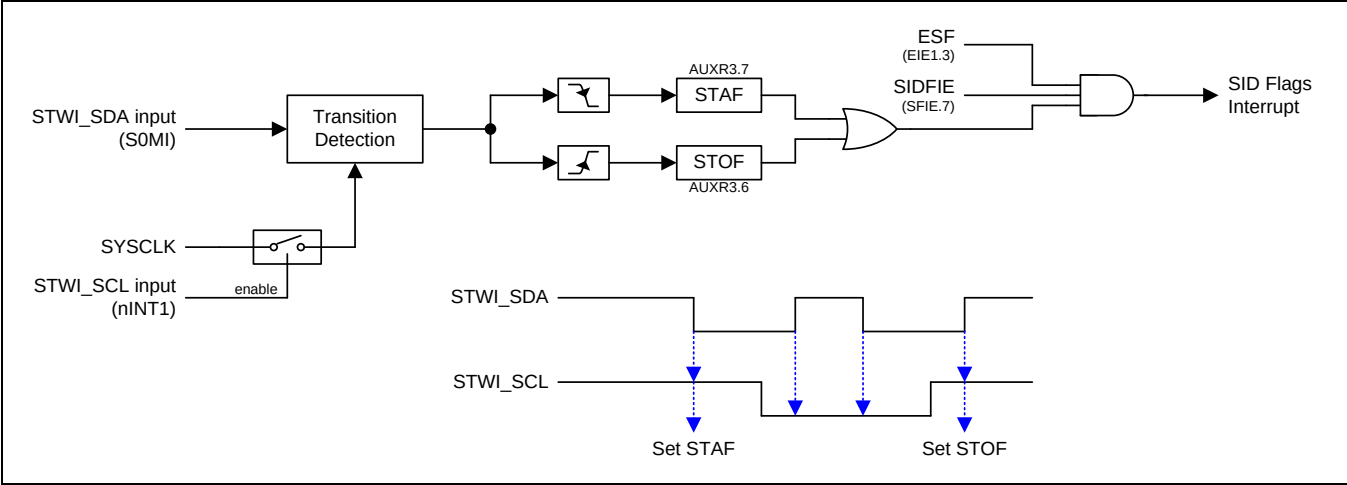
图 22-1.串行接口侦测结构
