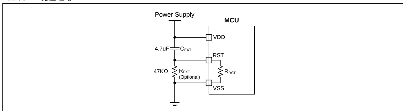
图 30-2. 复位电路
