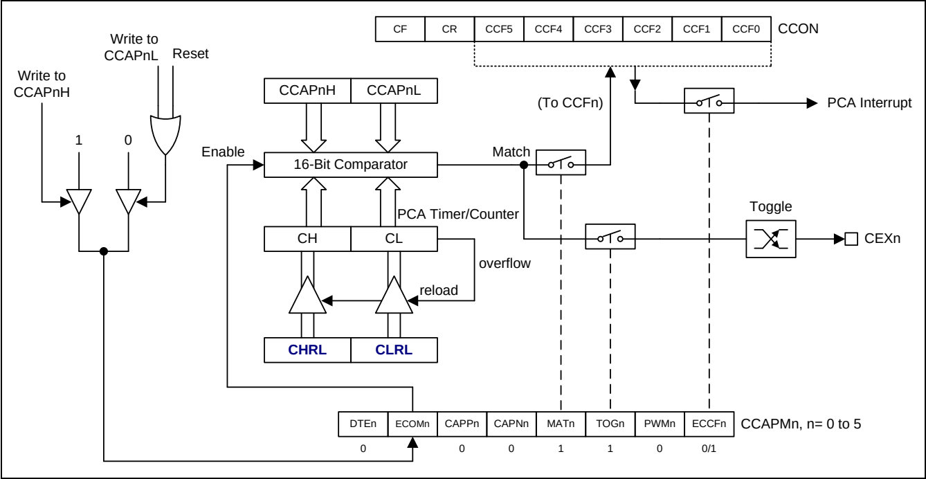
图 19–6. PCA 高速输出模式
