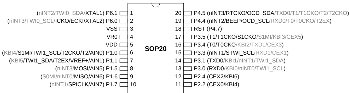
图 5-3. MA82G5BxxAS20 顶视图
