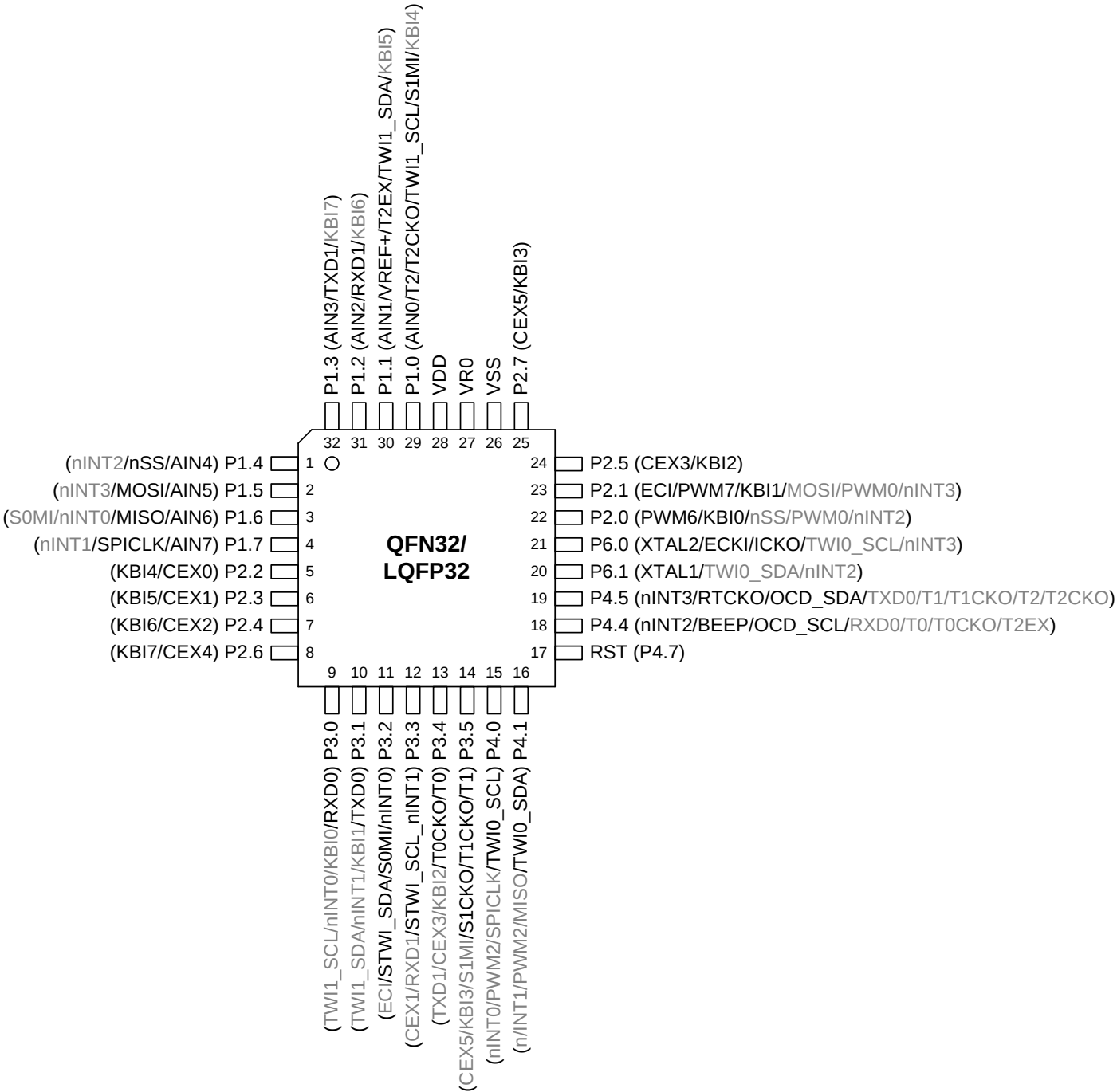
图 5-1. MA82G5BXXAD32 顶视图
