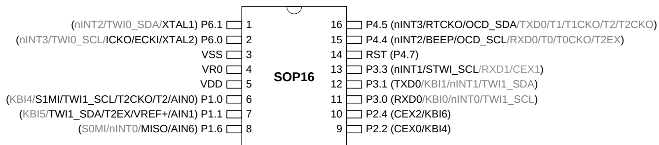
图 5-4. MA82G5BxxAS16 顶视图
