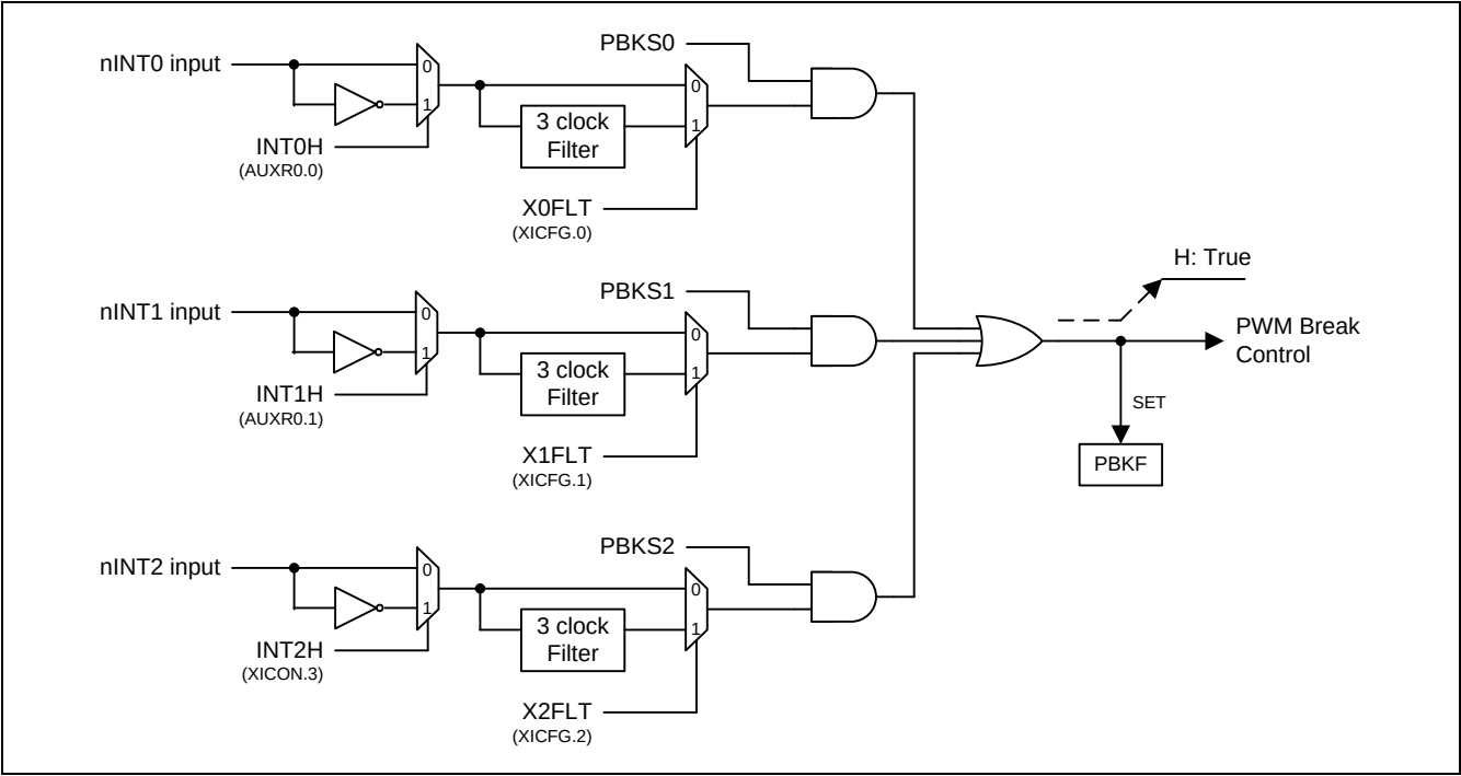
图 19–13. PWM 终止源
