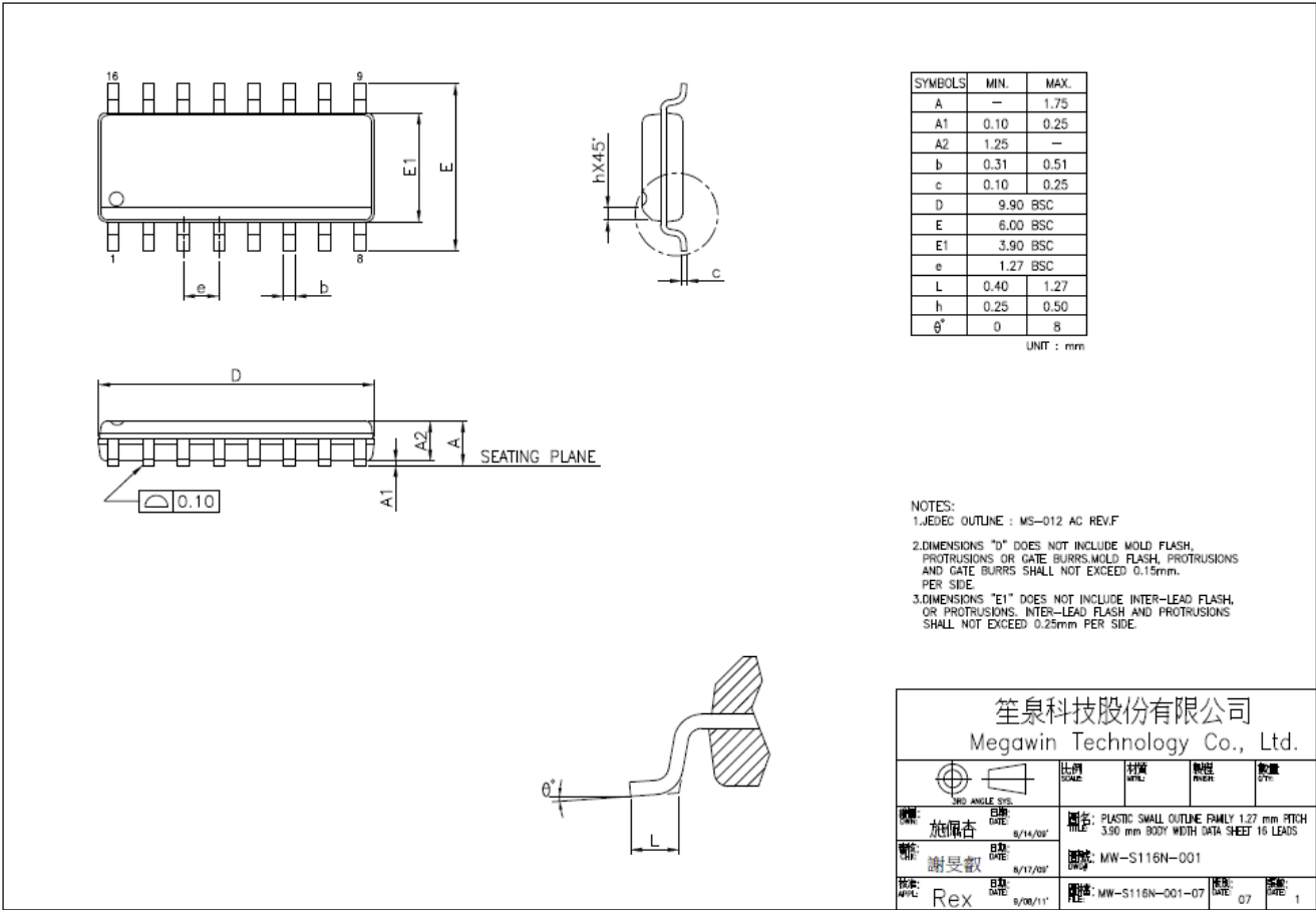
图 33-4. SOP-16(150mil)
