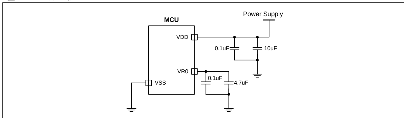
图 30-1. 电源电路
