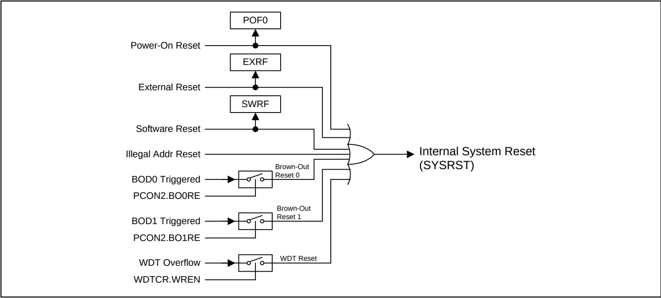
图 12-1. 系统复位源
