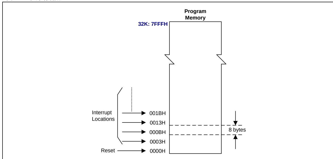
图 7-1. 程序存储器
