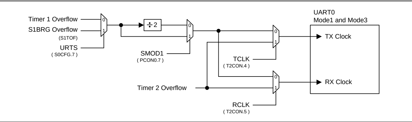
图 18-8. UART0 额外波特率源
