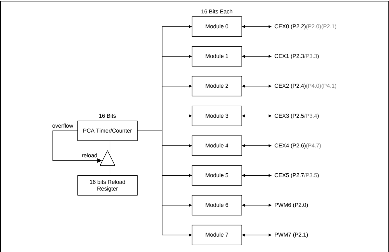
图 19-1. PCA 方框图
