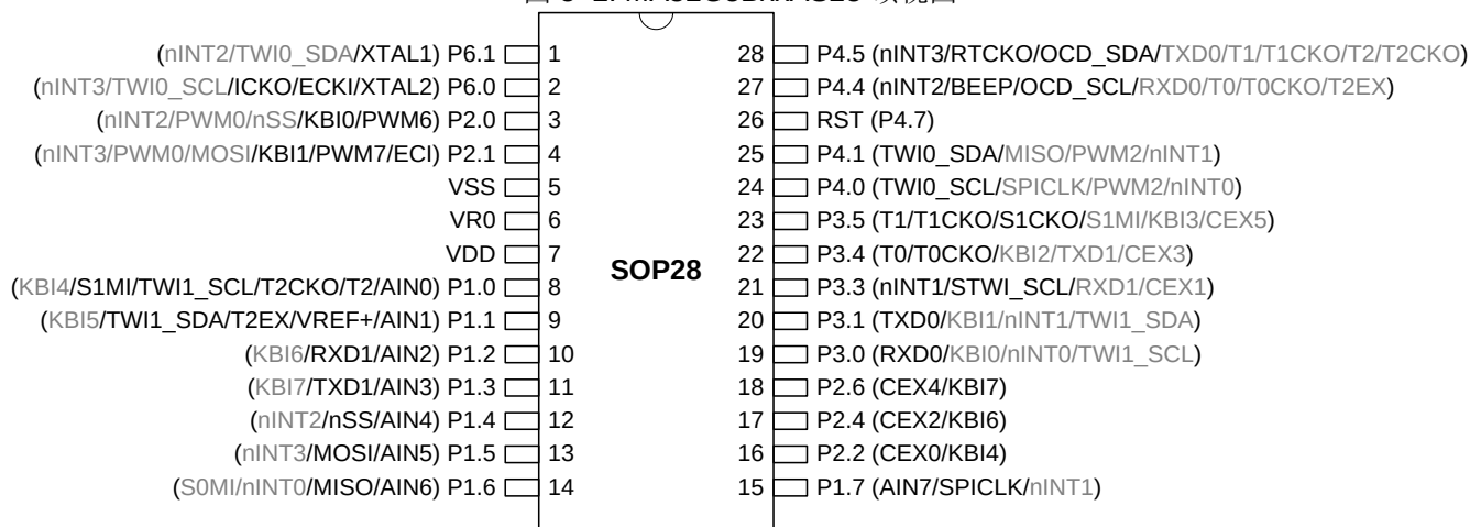
图 5-2. MA82G5BxxAS28 顶视图
