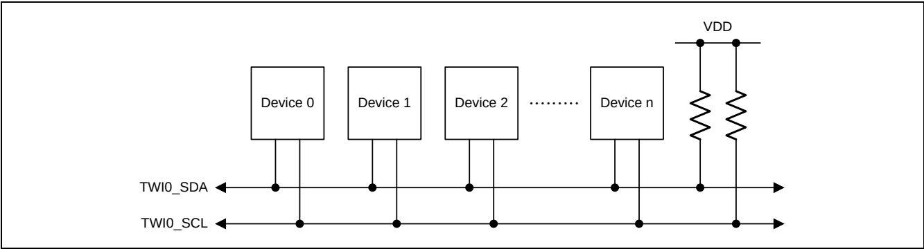
图 21-1. TWI0 总线互联框图
