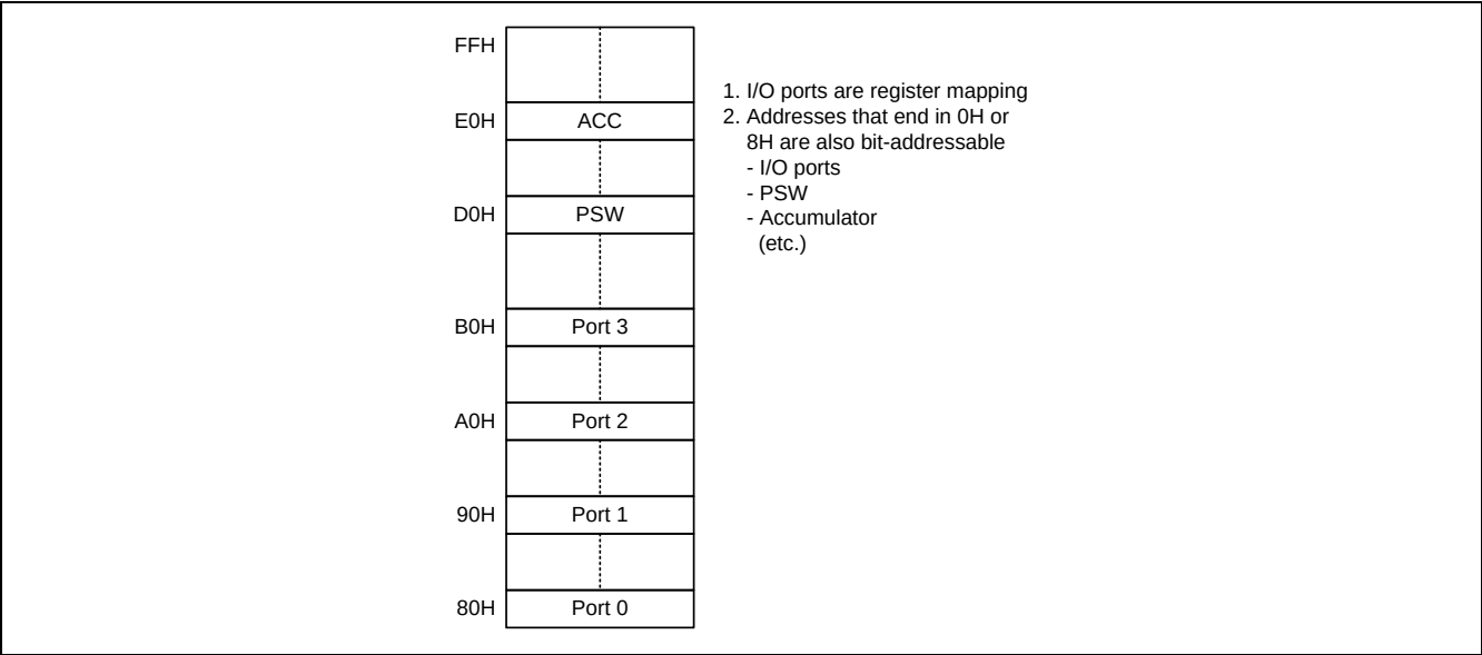
图 7-4. 特殊功能寄存器(SFR)空间
