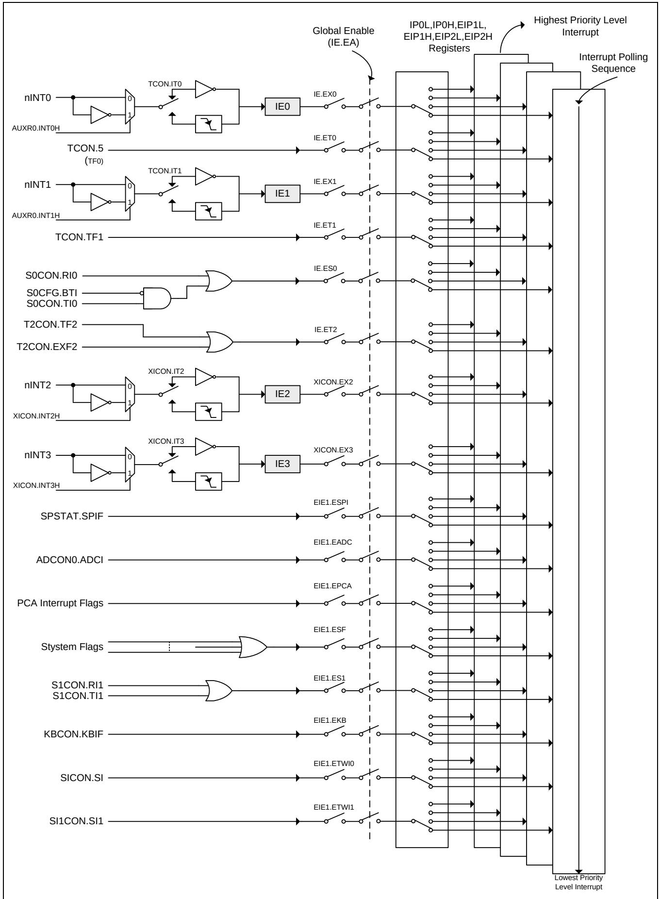
图 15-1. 中断系统
