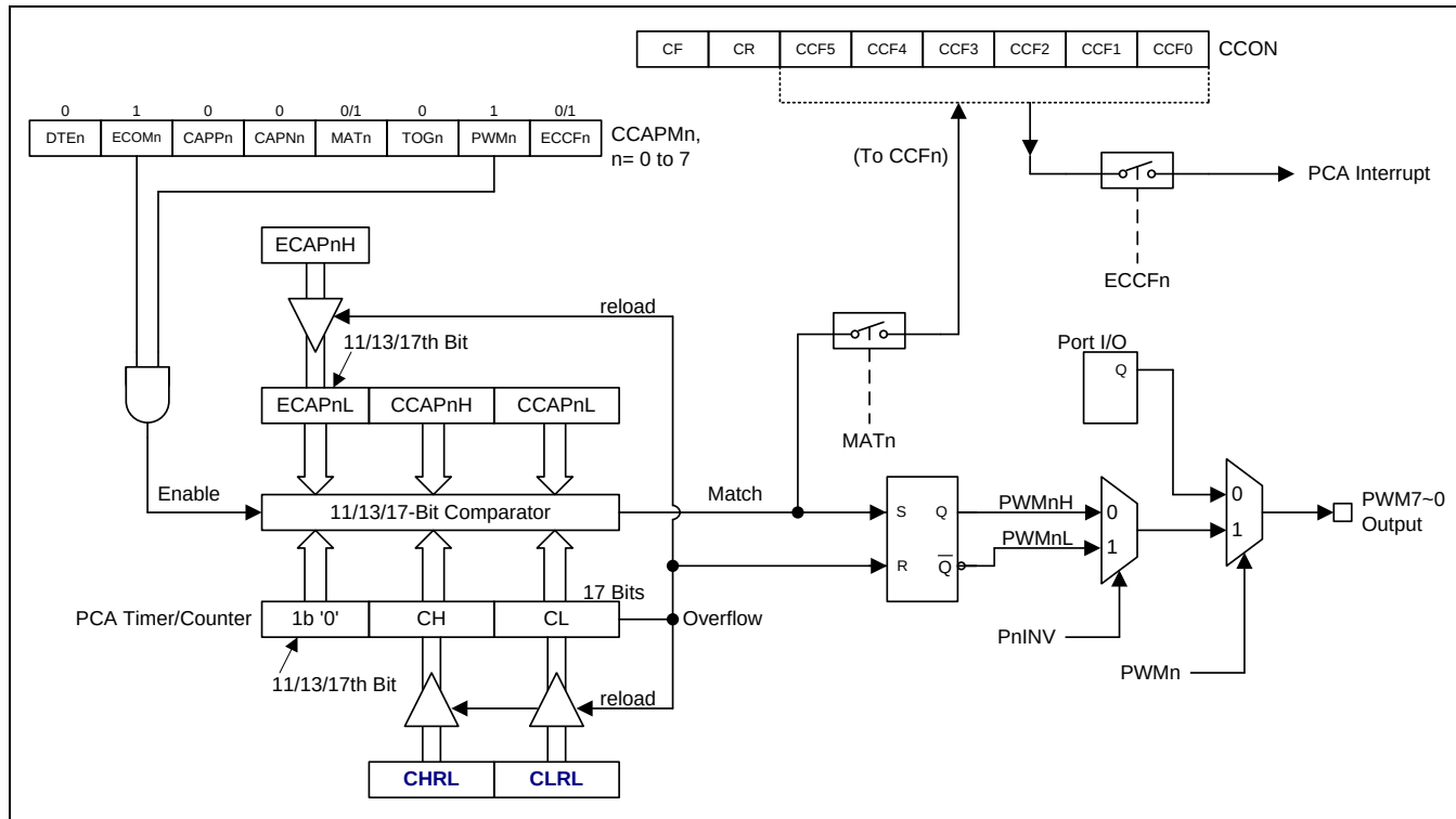
图 19-8. 10/12/16 位 PWM 模式的 PCA 增强型 PWM
