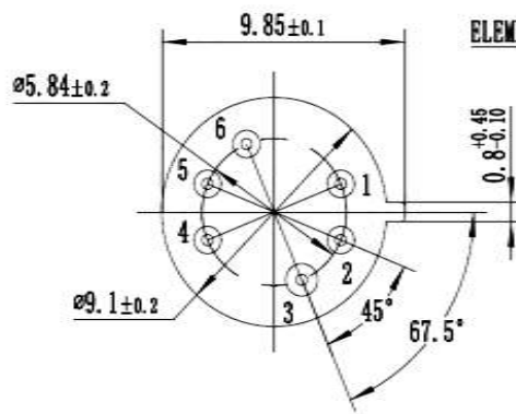
底视图
