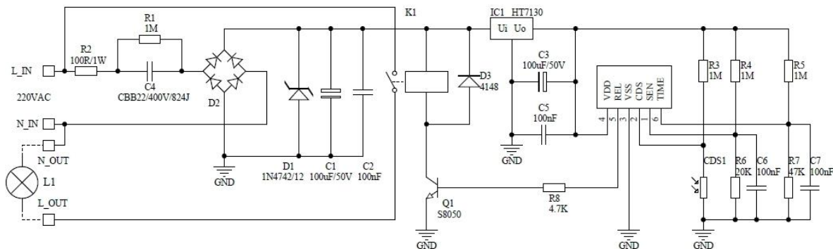
SY-DP-36BPF数字热释电传感器典型参考电路
