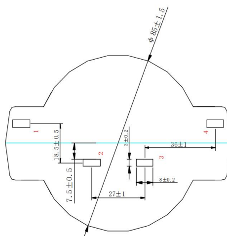
底视图
