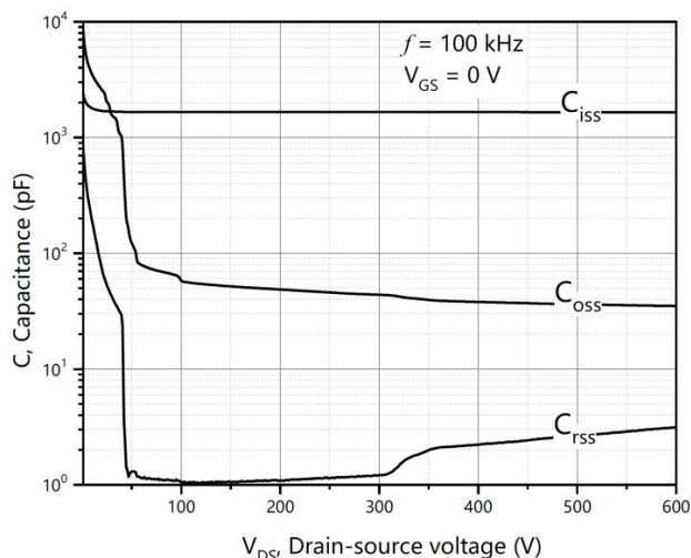
Typ. capacitances
