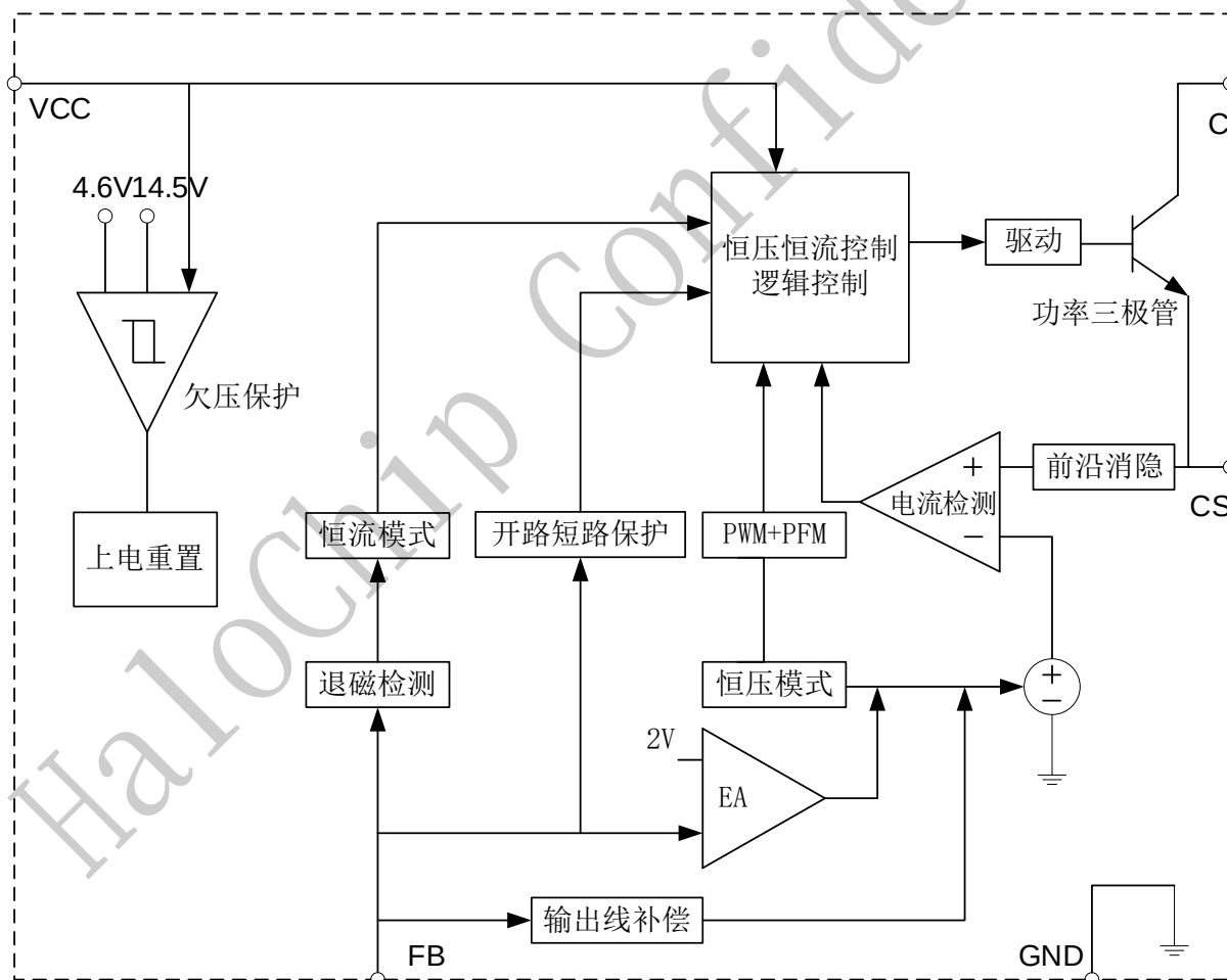
图 3 GP8611X 内部框图
