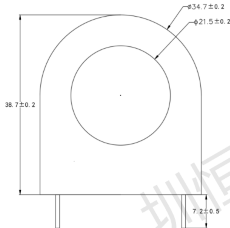
主视图
