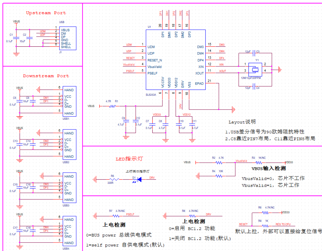
图 6: SL6243A 参考电路
