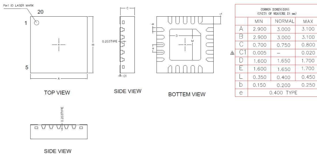
图 5: QFN20 封装尺寸图
