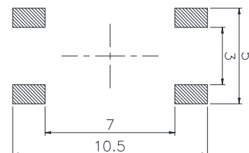
PCB. 焊接图
