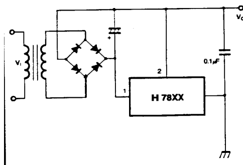
图 12、负输出电压电路
