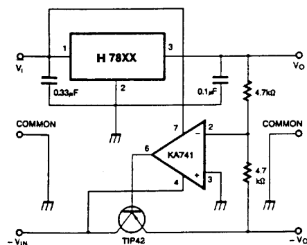
图 10、跟踪稳压器
