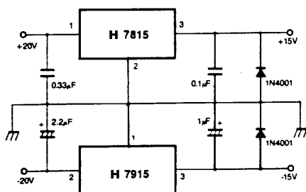
图 11、分离电源(±15V-1A)
