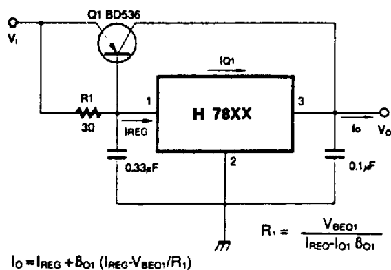
图 8、大电流稳压器
