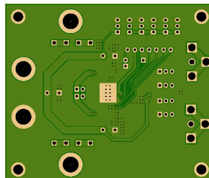
Fig 22-PCB Bottom Layer
