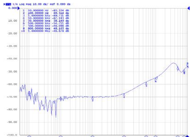
PSRR
