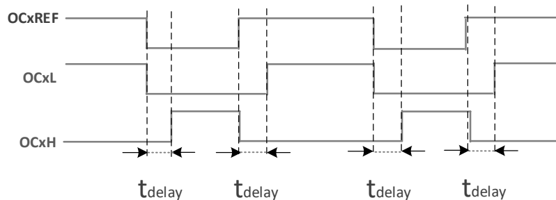
图 15-4 带死区插入的互补输出
