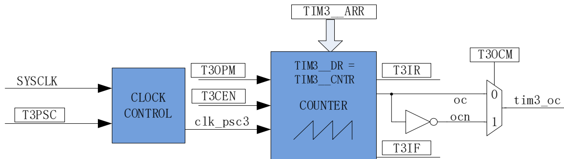
图 12-1 输出模式原理框图
