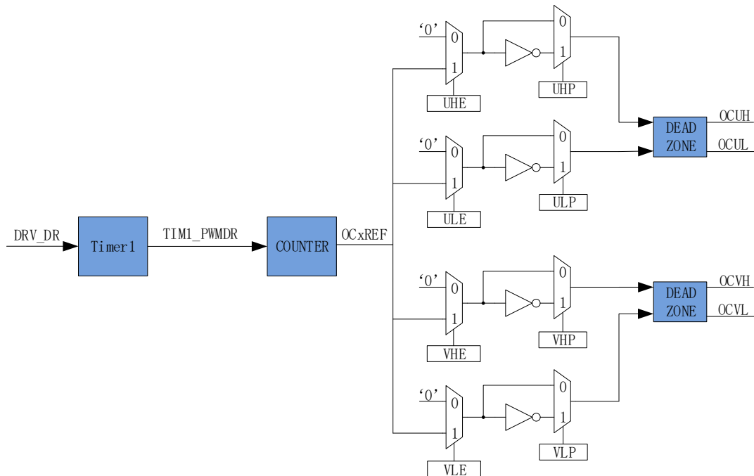
图 15-2 输出控制模块前级框图
