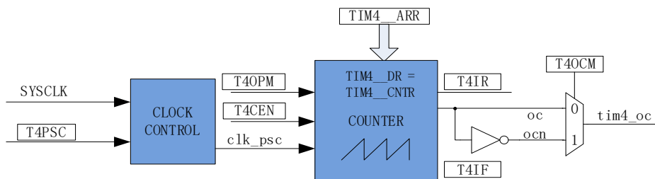
图 13-1 输出模式原理框图
