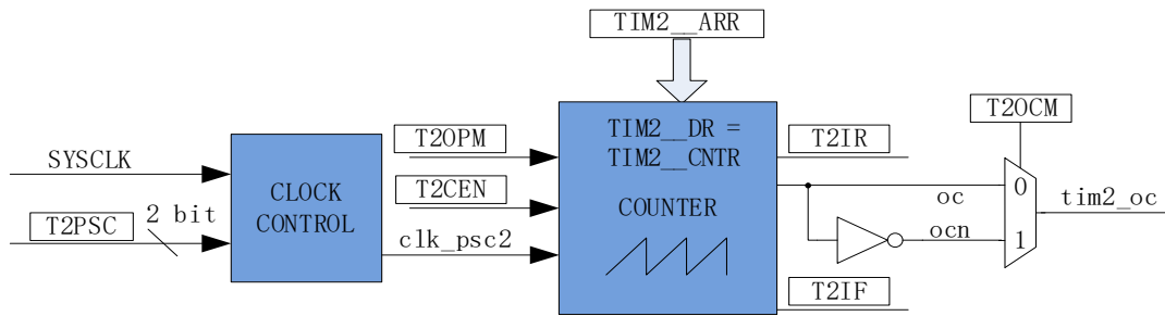
图 11-1 输出模式原理框图
