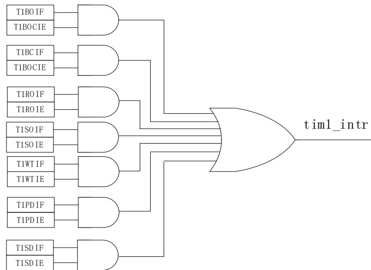
图 10-6 Timer1 中断源
