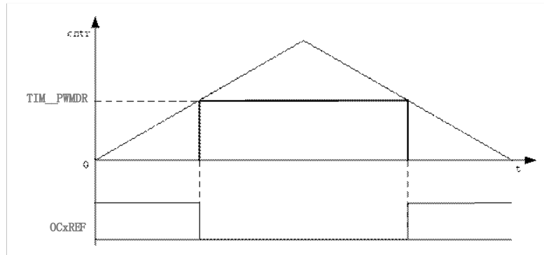
图 15-3 PWM 生成图
