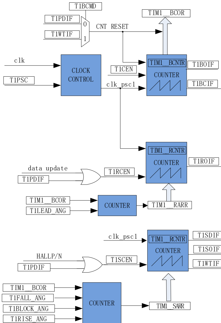
图 10-1 时基单元
