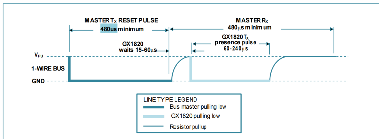
Figure13.初始化时序
