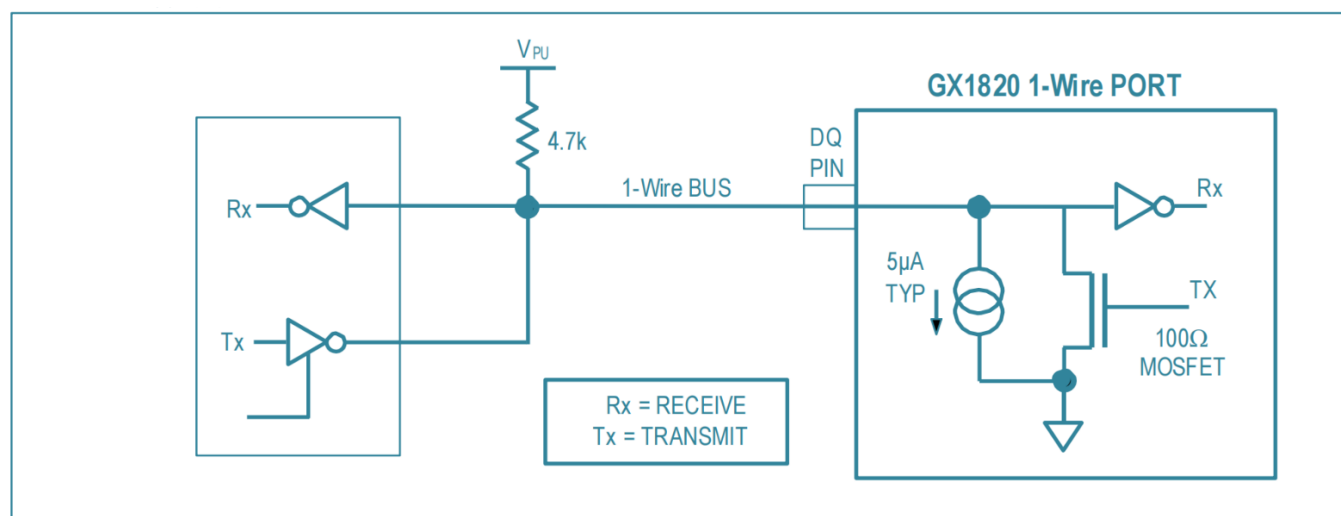
图10.硬件结构图
