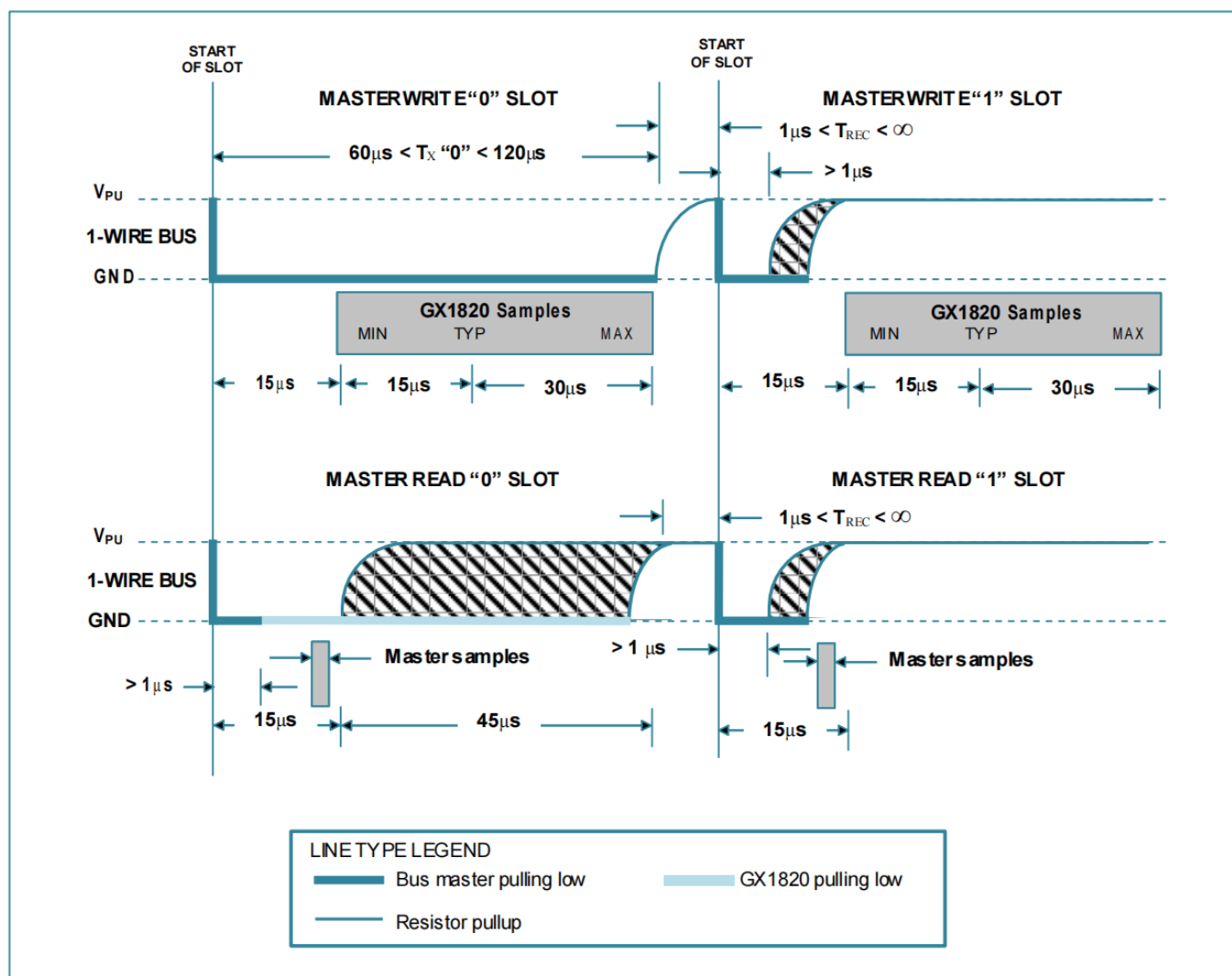
Figure14.Read/WriteTimeSlotTimingDiagram
