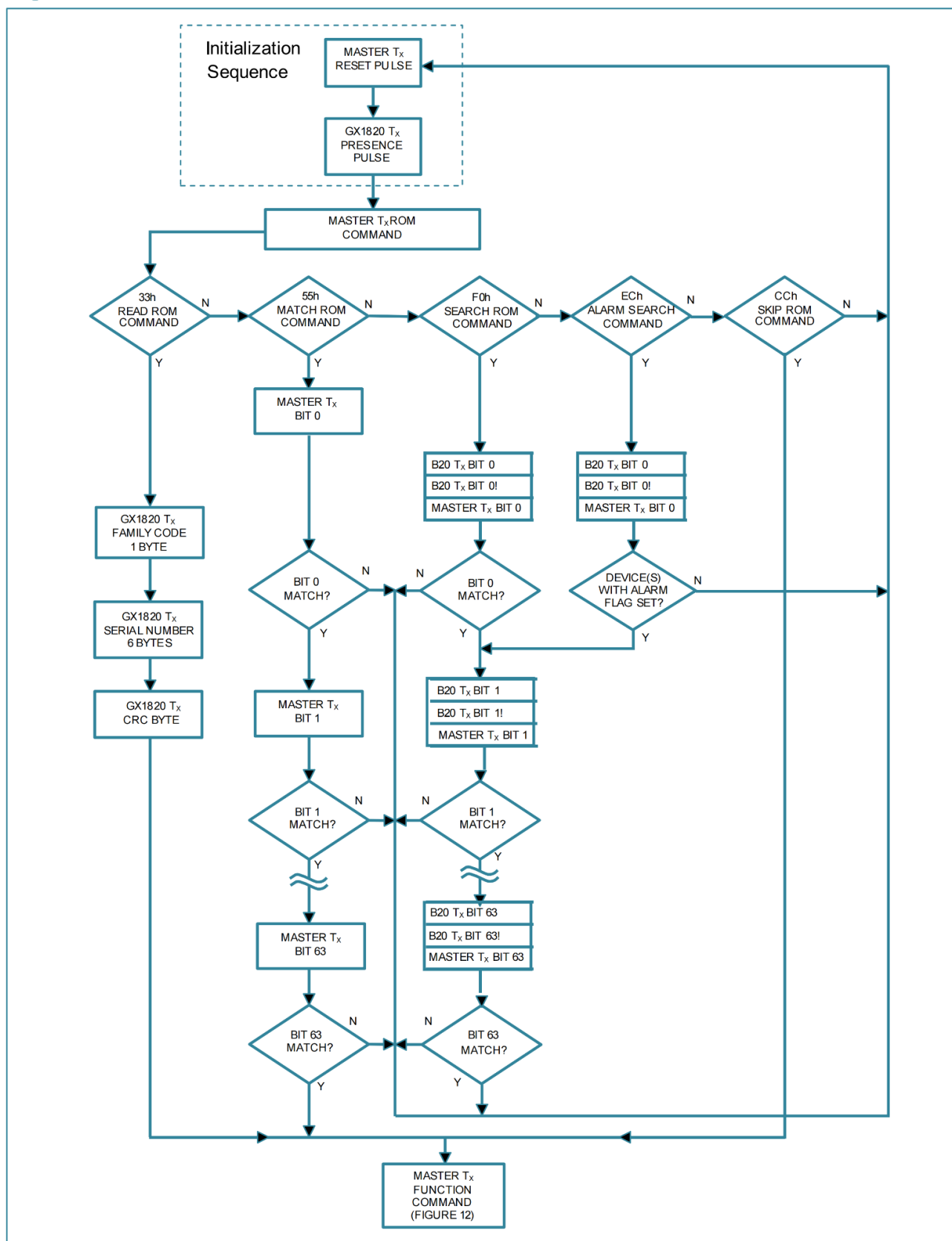
Figure11. ROM指令流程图
