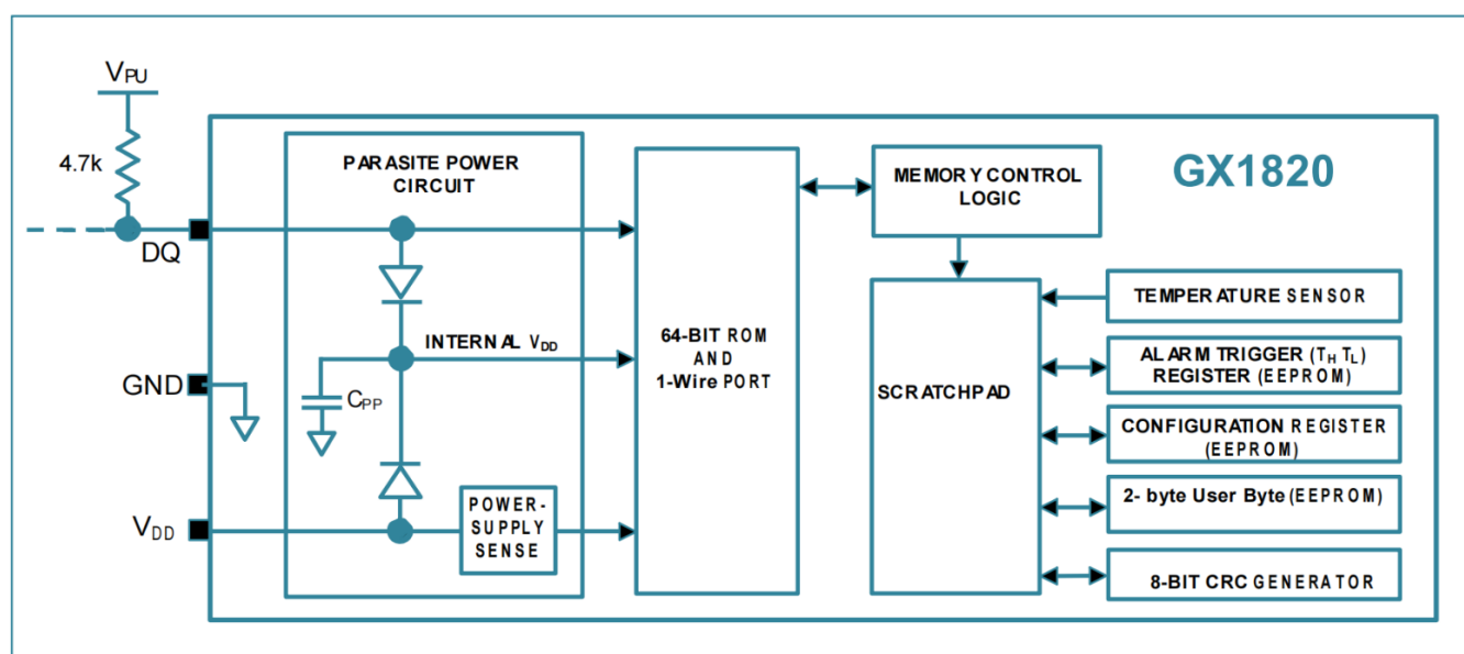
图1. GX1820的结构框图
