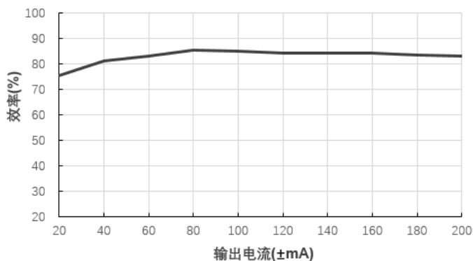
效率Vs输出电流(Vin=12V)@E1205S-2WR2
