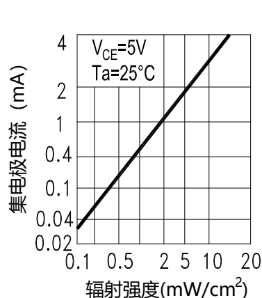
图五：集电极电流VS辐射照度
