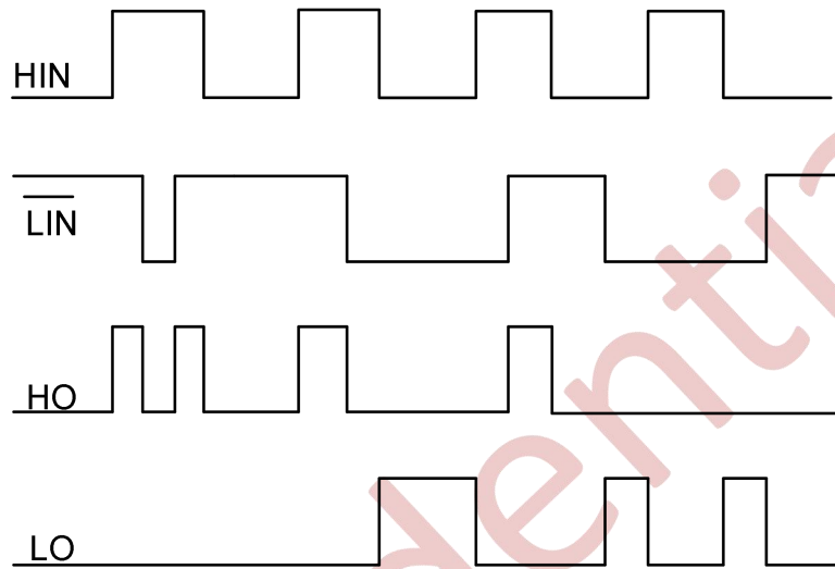
图 9-1 NSG6004 输入输出时序波形
