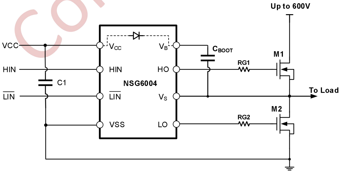
图 10-2 NSG6004 典型应用电路图
