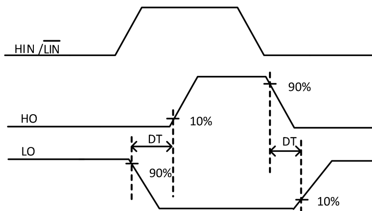
图 9-3 防直通延时波形定义
