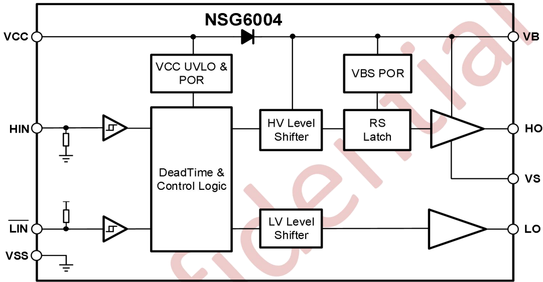
图 10-1 NSG6004 的功能框图
