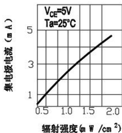
图五：集电极电流VS辐射照度
