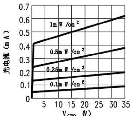
图六：光电流VS V_{CE0} 曲线
