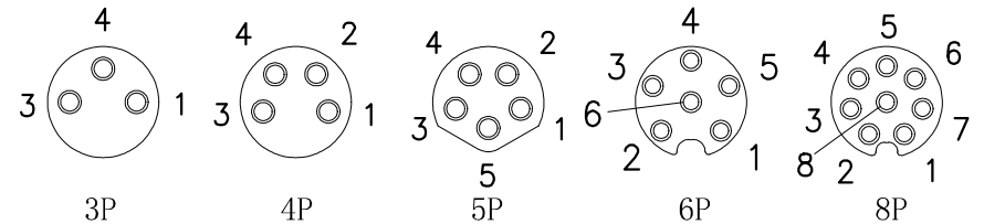
PIN位分布(前视图)
