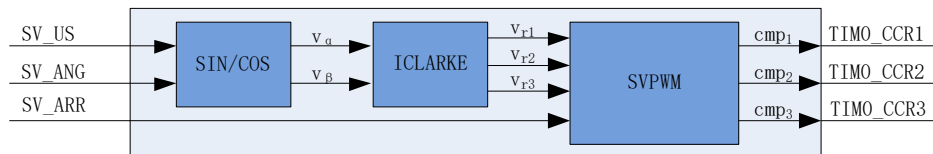
图 14-1 SVPWM 原理框图
