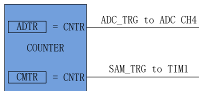
图 18-3 TIMER2 的 ADC 触发和比较器采样功能
