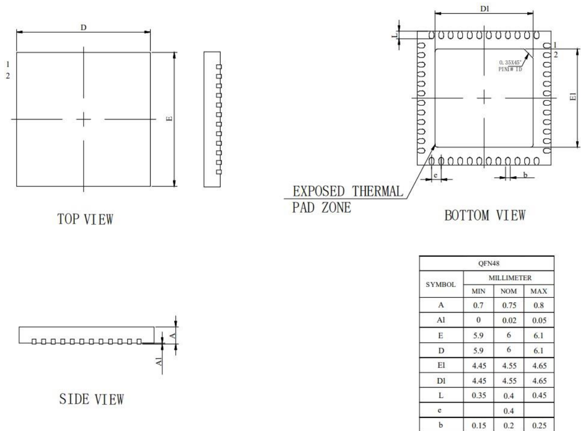
图 3-3 QFN48_6X6 封装尺寸图选项二
