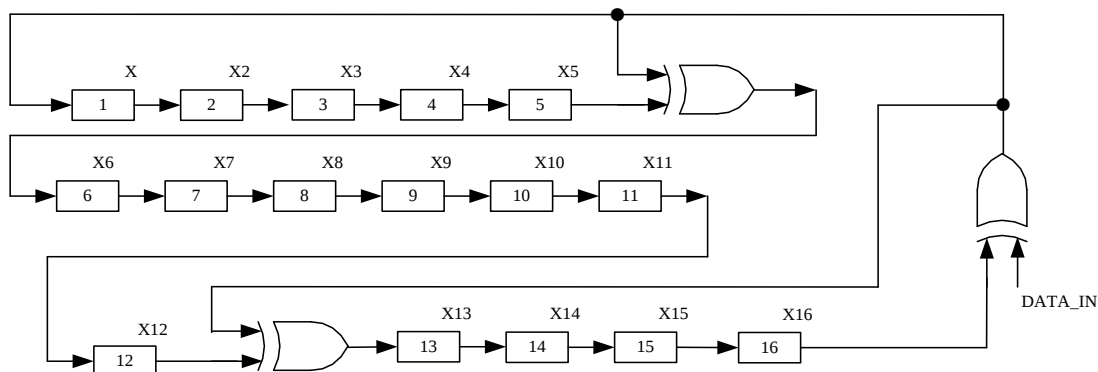
图 32-1 CRC16 电路原理图
