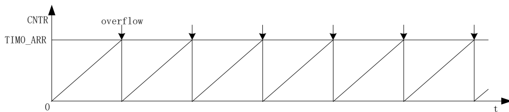
图 16-3 边沿对齐向上计数模式
