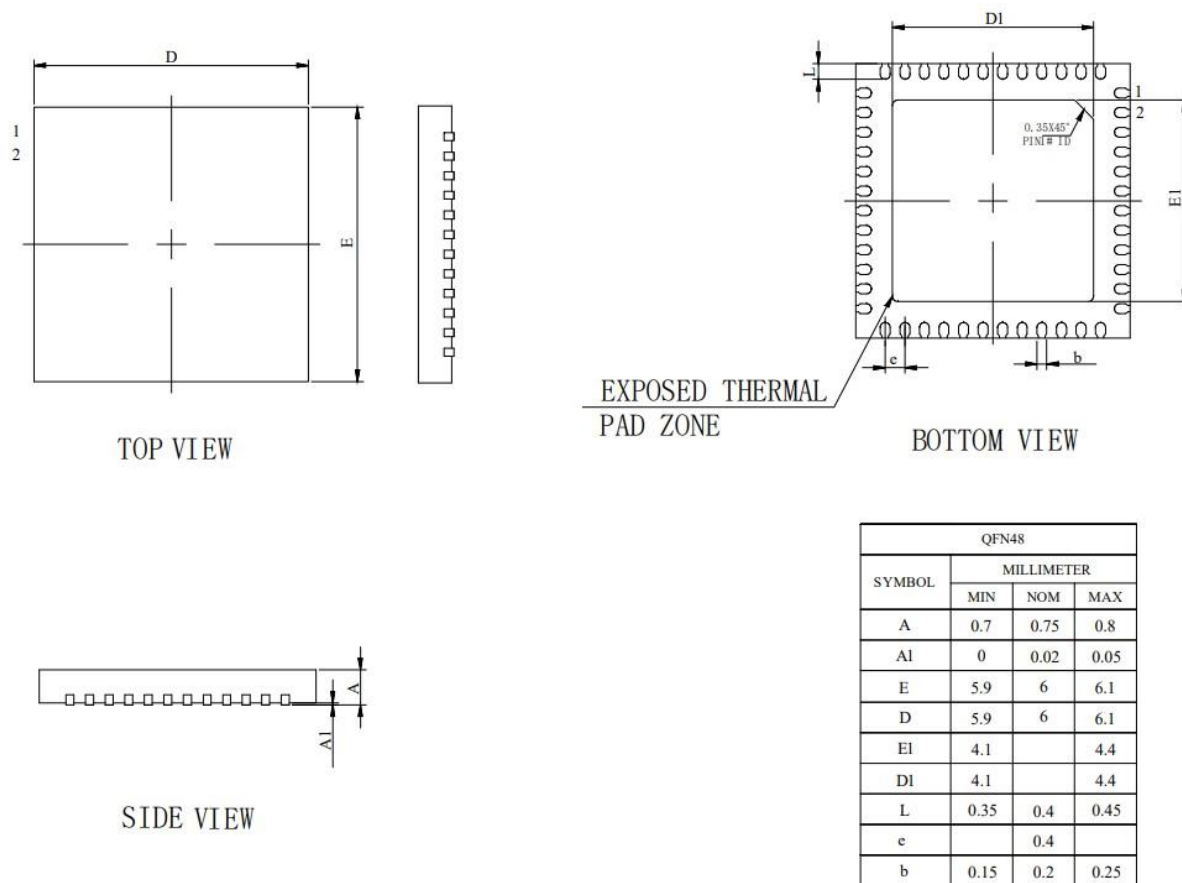
图 3-2 QFN48_6X6 封装尺寸图选项一
