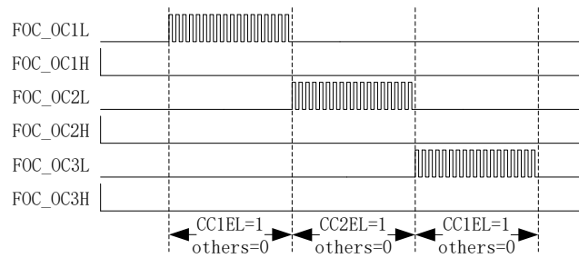
图 15-18 预充电图
