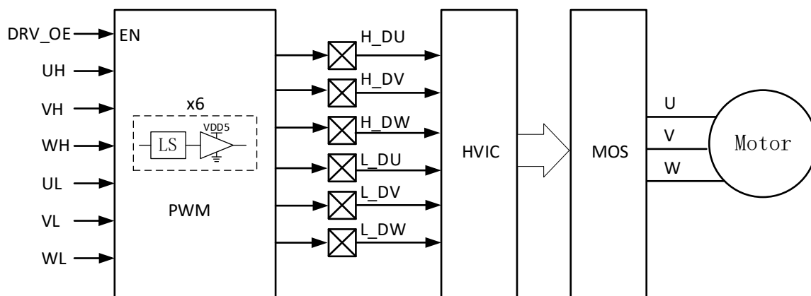
图 29-2 PWM 模式的原理图
