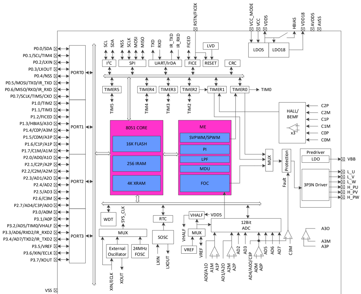
图 1-3 FU6831N 功能框图
