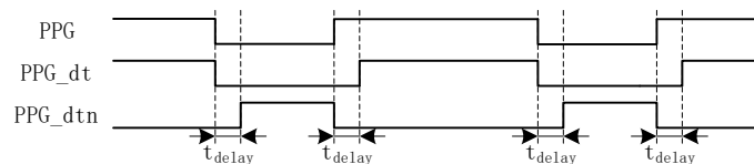
图 17-14 带死区插入的互补输出
