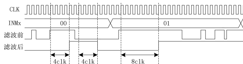
图 17-6 滤波模块时序图
