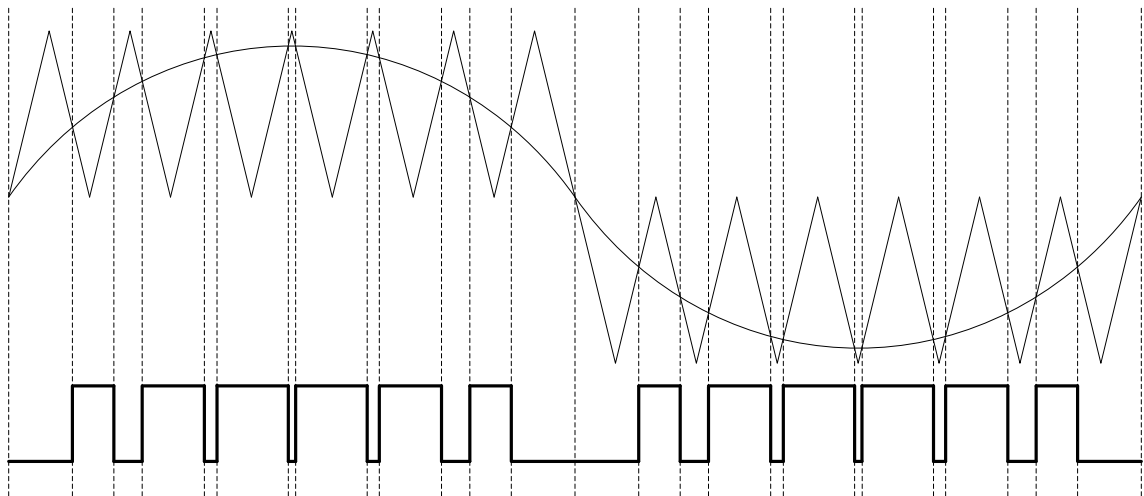
图 14-6 单极性 SPWM
