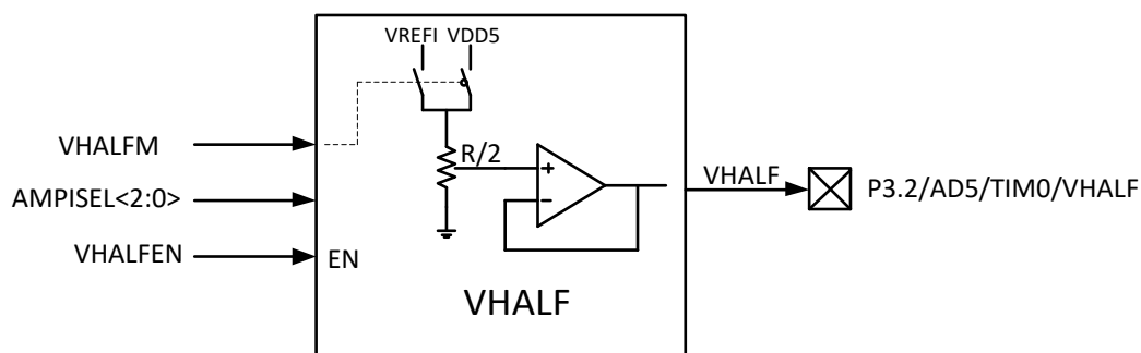
图 26-1 VHALF 模块的端口输入输出情况
