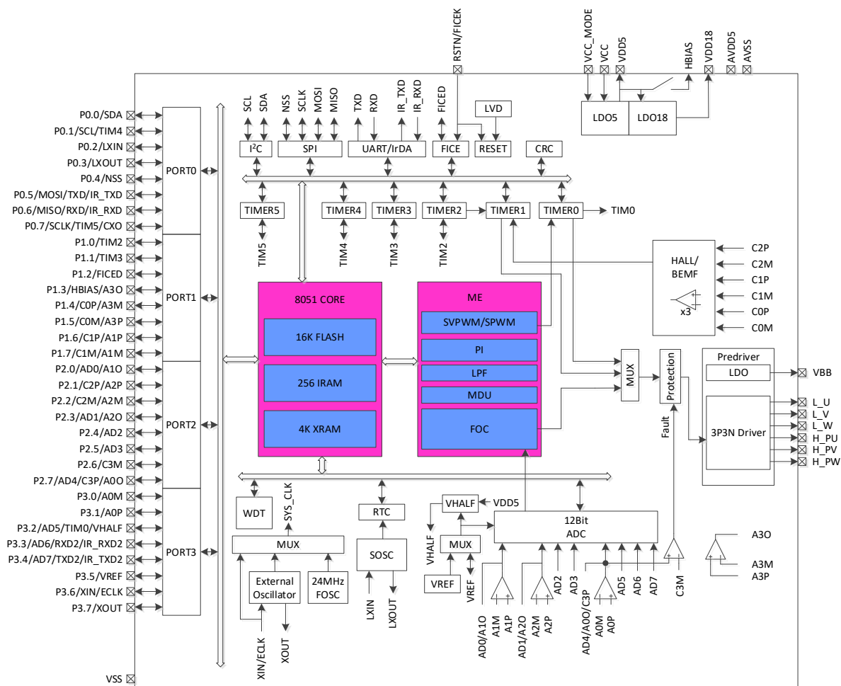
图 1-2 FU6831Q 功能框图
