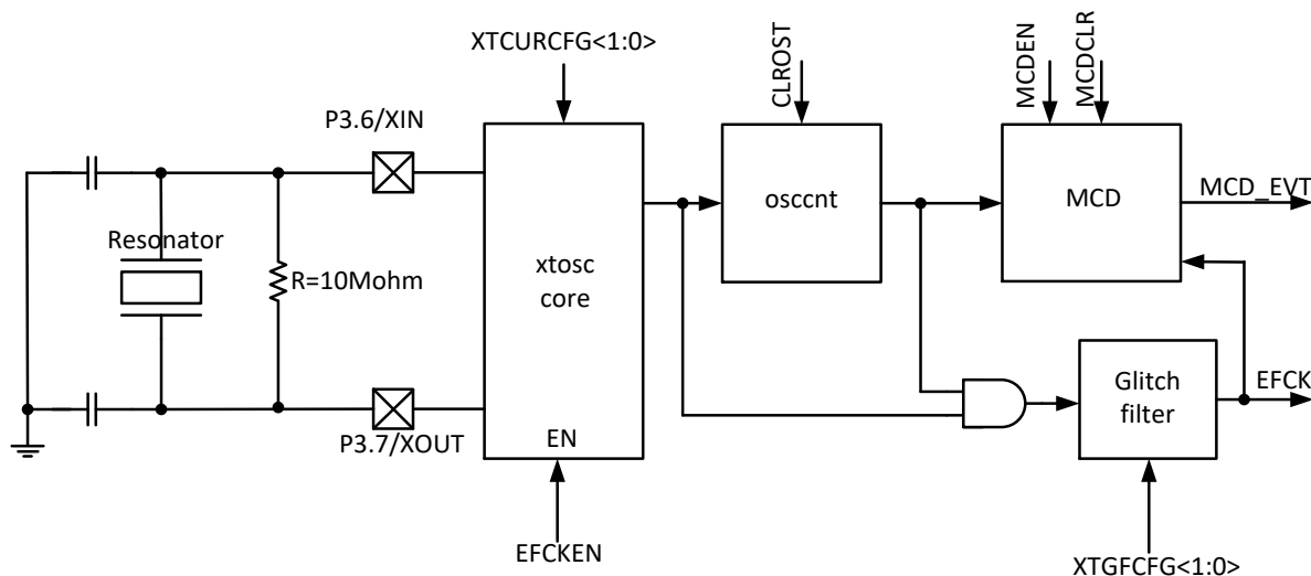
图 22-1 外部快时钟 xtosc 模块晶体输入模式
