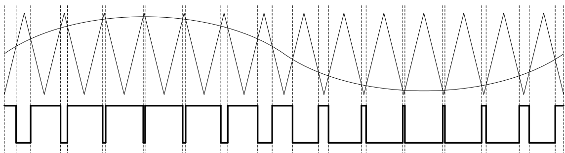
图 14-7 双极性 SPWM
