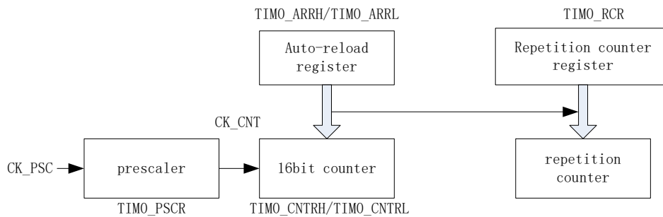
图 16-2 时基单元
