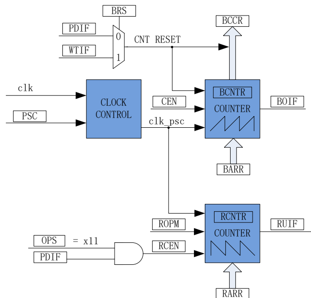
图 17-2 时基单元
