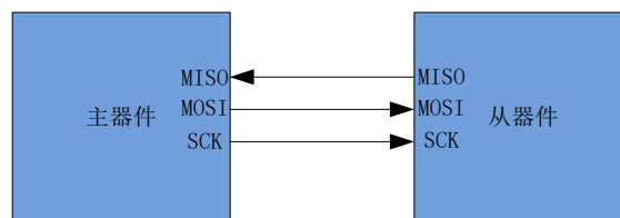
图 9-2 3 线单主方式和 3 线单从方式连接图
