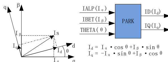
图 15-5 PARK 变换
