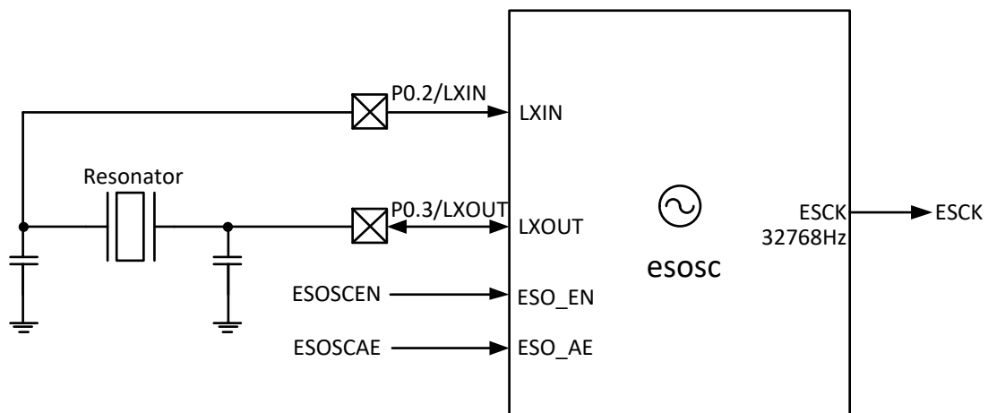
图 22-4 外部慢时钟 esosc 的端口输入输出情况
