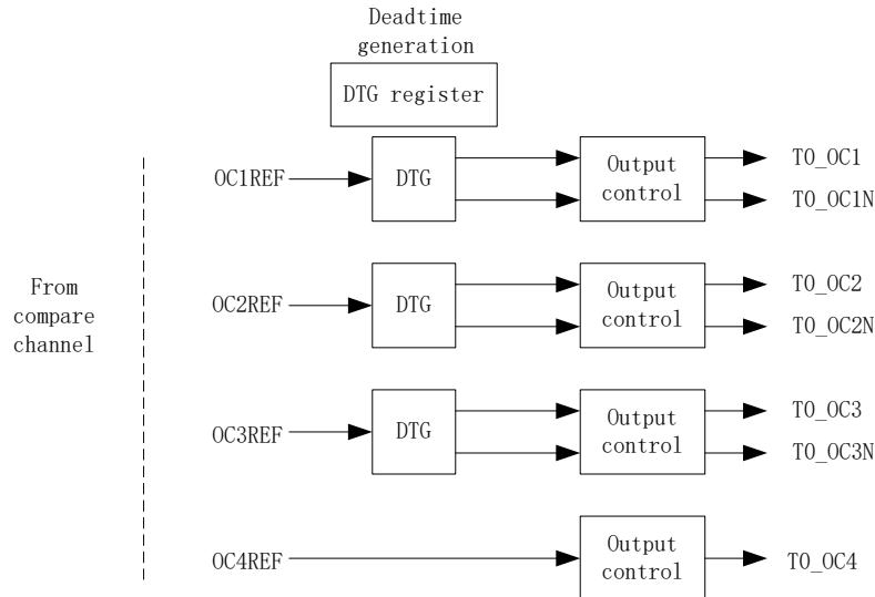
图 16-12 通道 4 输出模块框图
