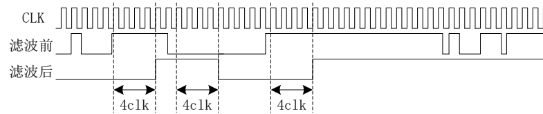
图 18-5 滤波模块时序图
