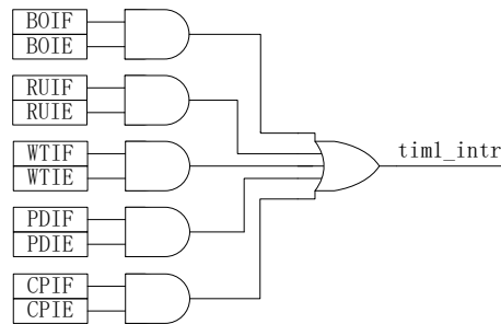
图 17-17TIMER1 中断源
