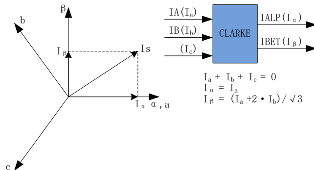
图 15-4 CLARKE 变换
