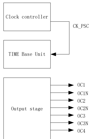
图 16-1 TIM0 框图
