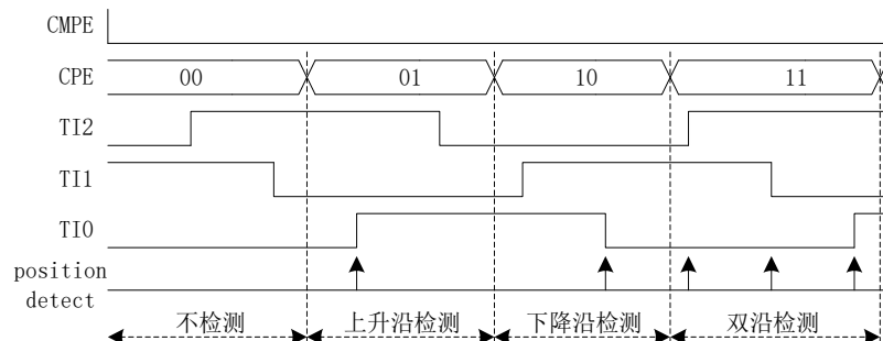
图 17-9 CMPE=0 位置检测时序图
