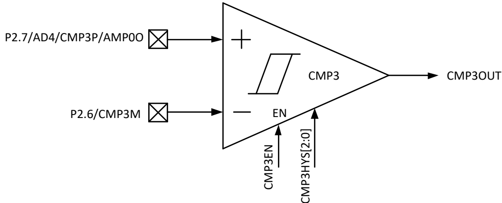
图 28-1 比较器 CMP3 的输入输出相关信号
