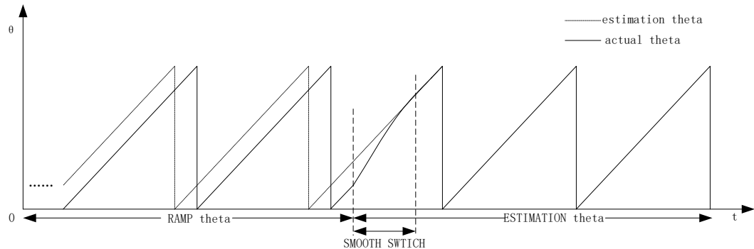
图 15-14 角度平滑切换曲线
