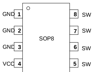
GP7596X 管脚封装图
