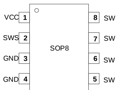
GP7596XA 管脚封装图
