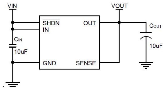
图 1 LKP41220S-1.8/3.3 典型应用电路图
