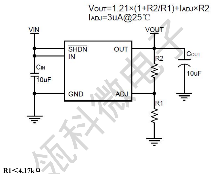
图 2 LKP41220S-ADJ 典型应用电路图
