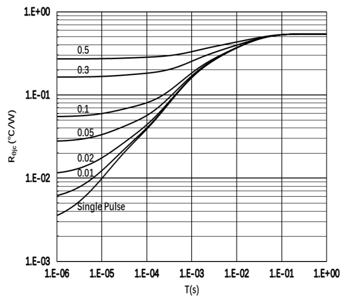
图 7 瞬态热阻抗
