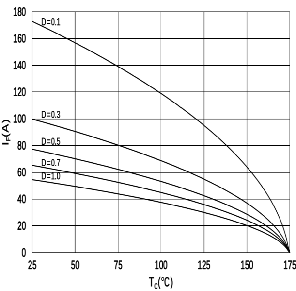
图 8 不同负载下的电流曲线
