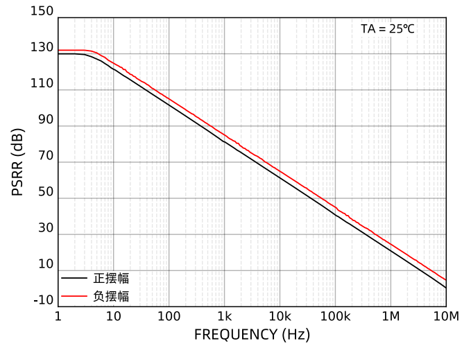
图 20 PSRR
