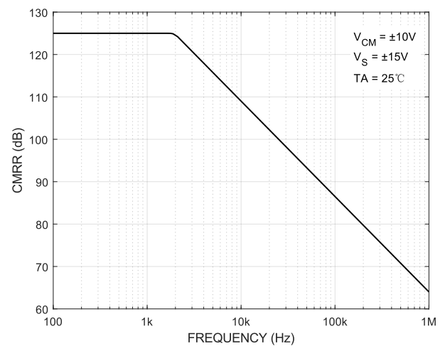
图 18 CMRR
