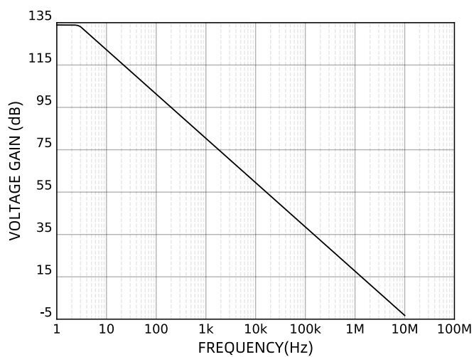
图 6 电压增益
