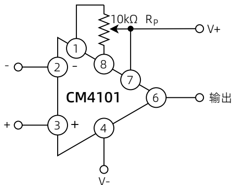
图 22 失调归零电路
