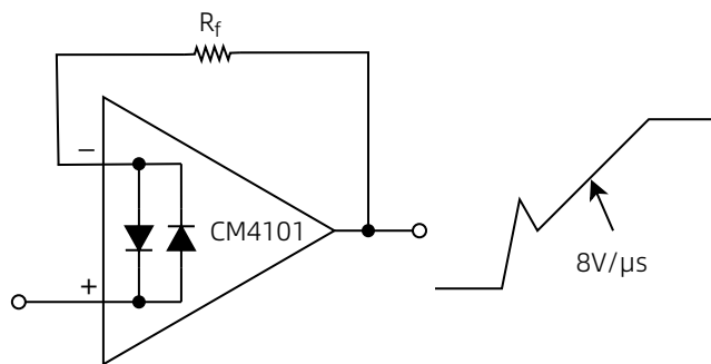
图 24 阶跃响应
