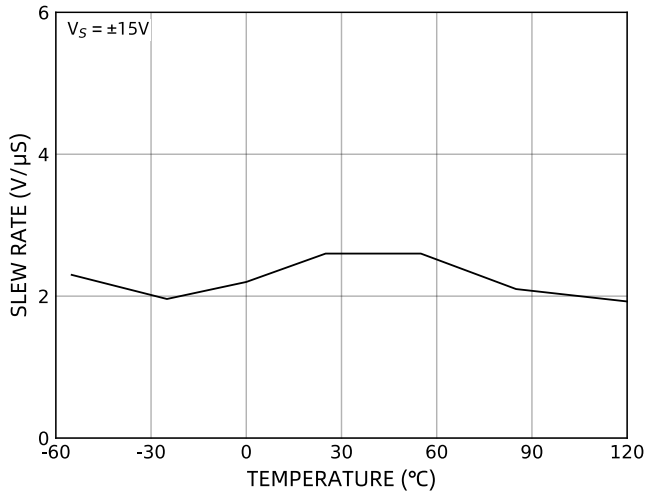
图 7 压摆率随温度的变化
