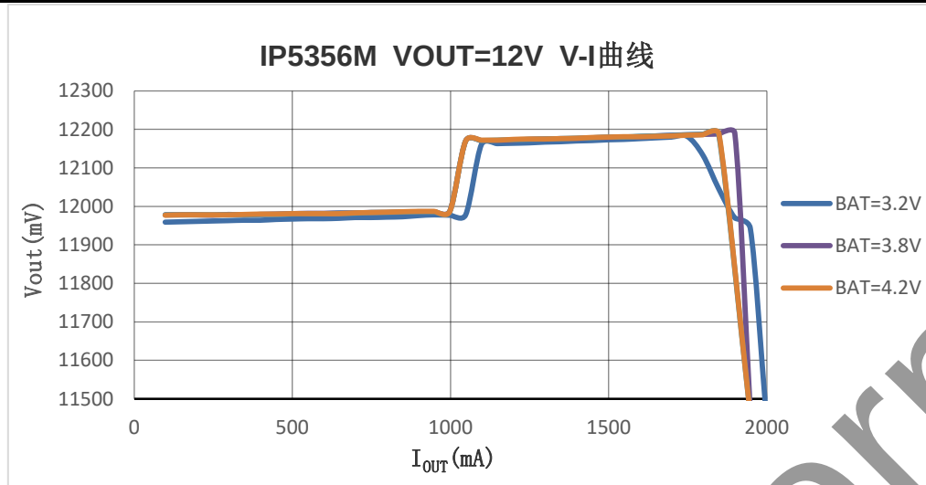
图 9 IP5356M VOUT=12V V-I 曲线
