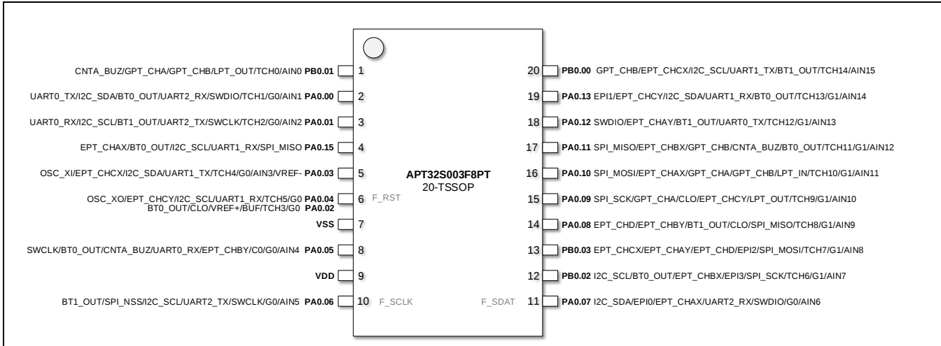
Figure 2-1 管脚定义图(20PIN) /PIN6有两个I/O的功能，但不能同时使用，请参考下页注释8。
