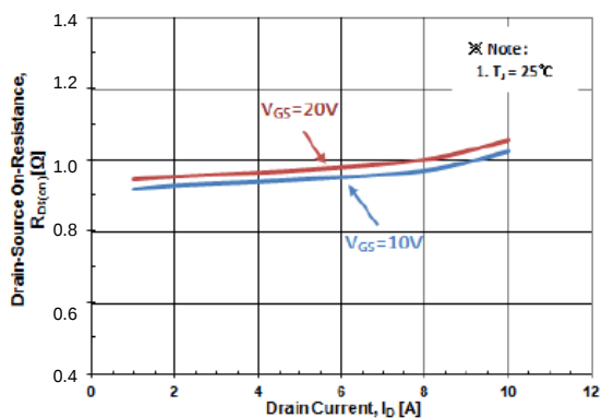
Fig. 3 R_{DS(ON)} - I_D
