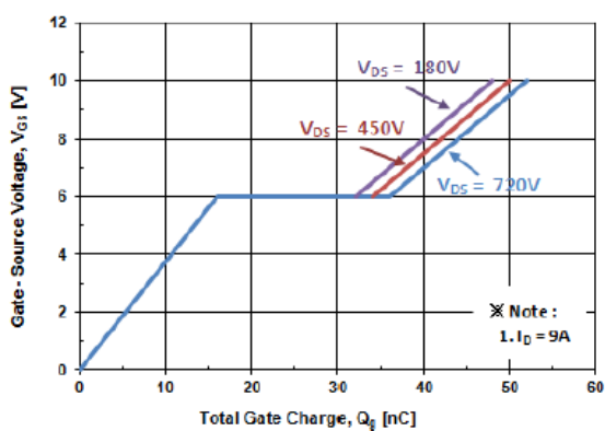
Fig. 6 V_{GS} - Q_G
