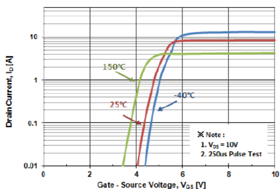
Fig. 2 I_D - V_{GS}
