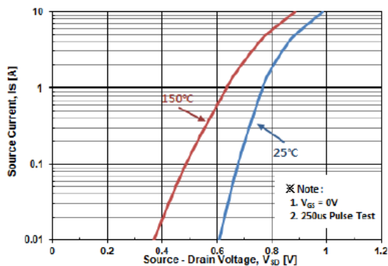
Fig. 4 I_S - V_{SD}
