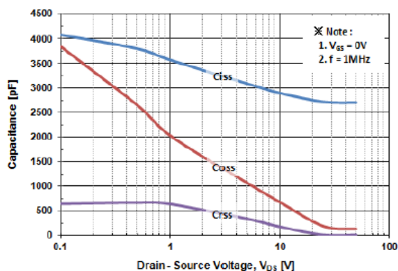
Fig. 5 Capacitance - V_{DS}
