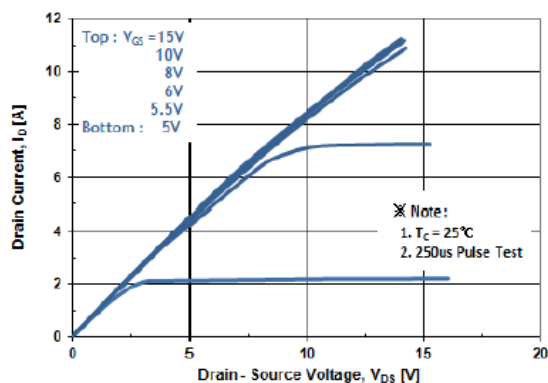
Fig. 1 I_D - V_{DS}
