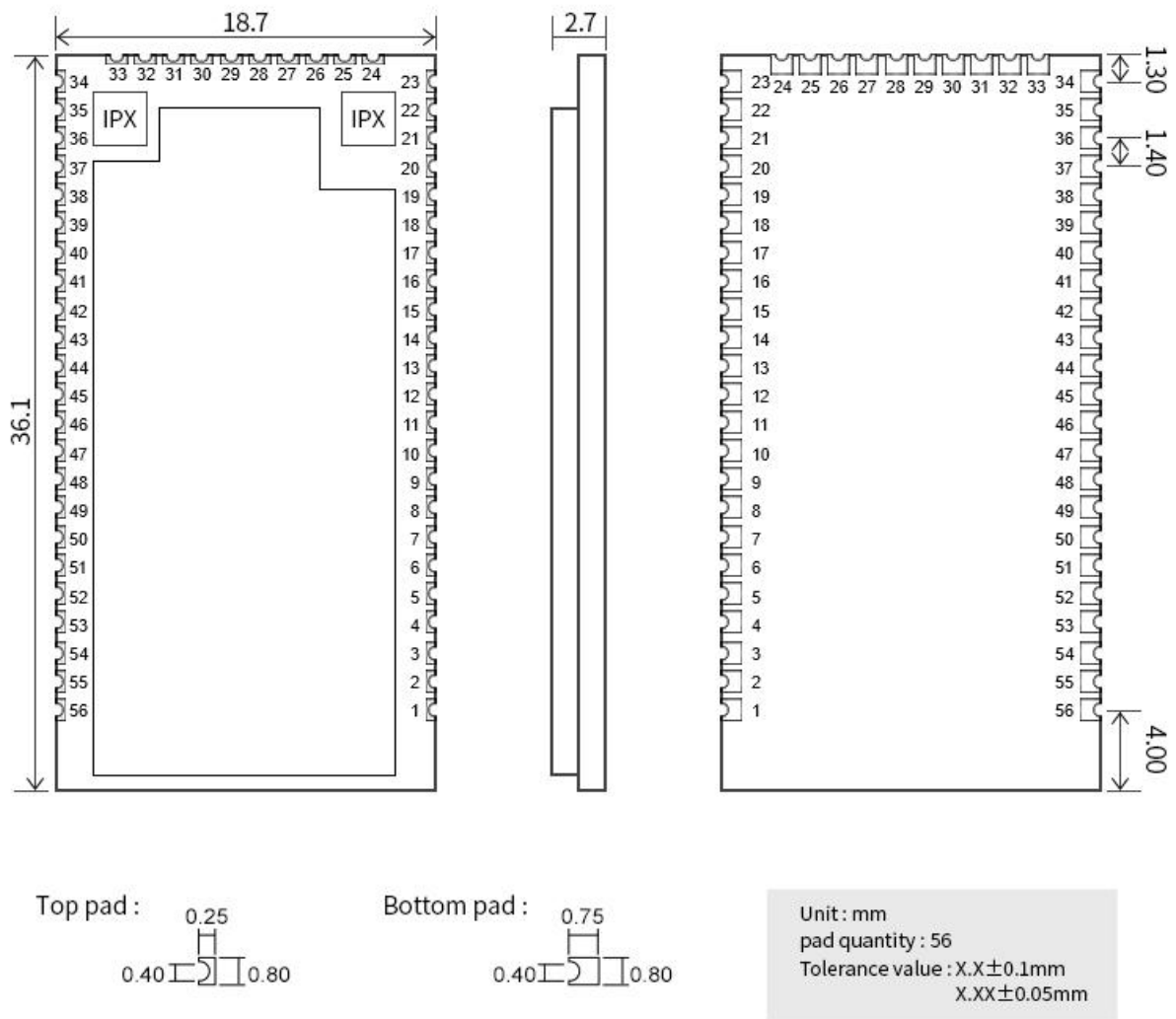
Figure 2 : Dimensions of E103-W20(7628)
