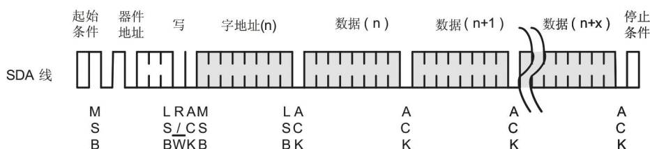
图10页写
