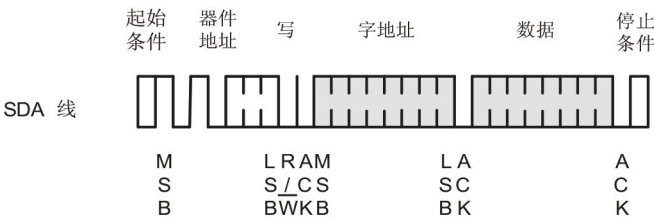
图9 字节写
