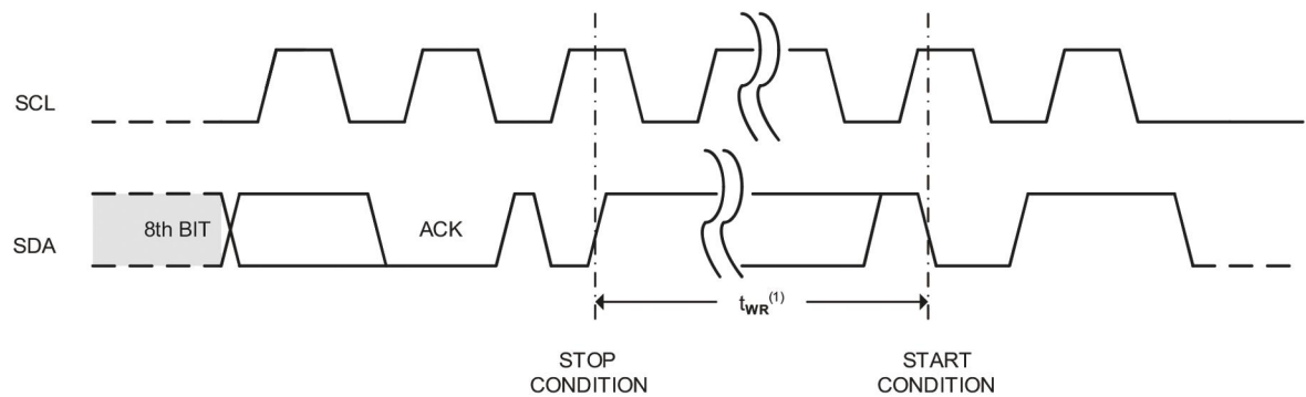
图2 总线时序
