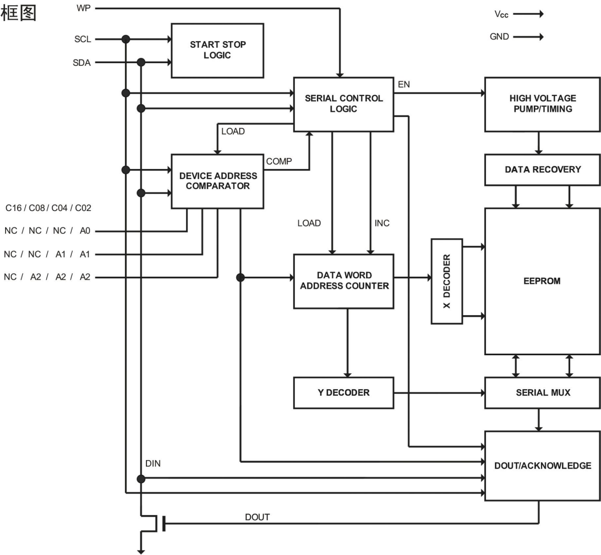
图1 框图
