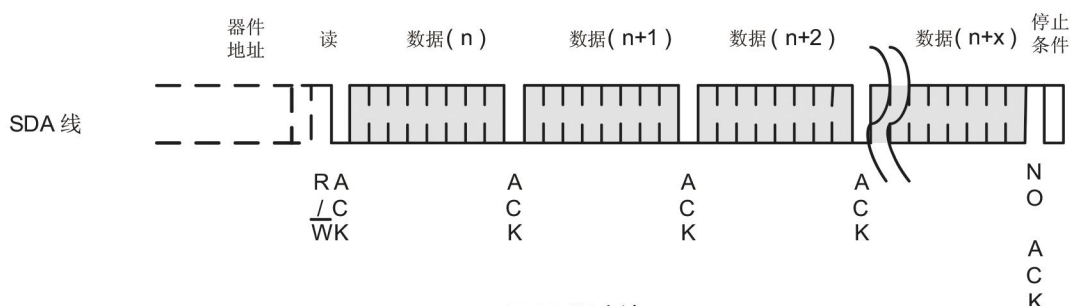
图14 顺序读
