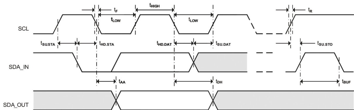
图2 总线时序
