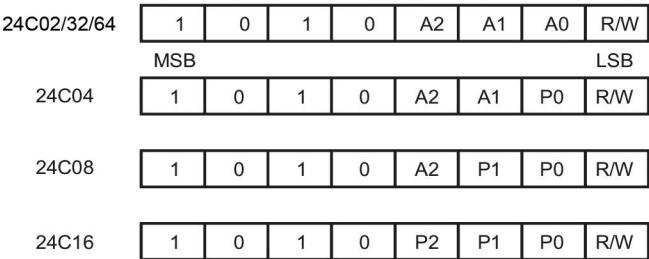
图8 器件地址
