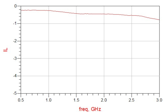
Figure 10. MHC0530W03 IL
