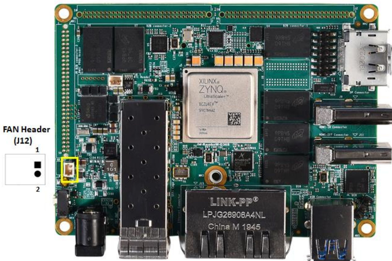
Figure 15: Fan Header
