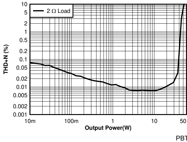
图 7-37. THD+N vs Power - PBTL - 384kHz
