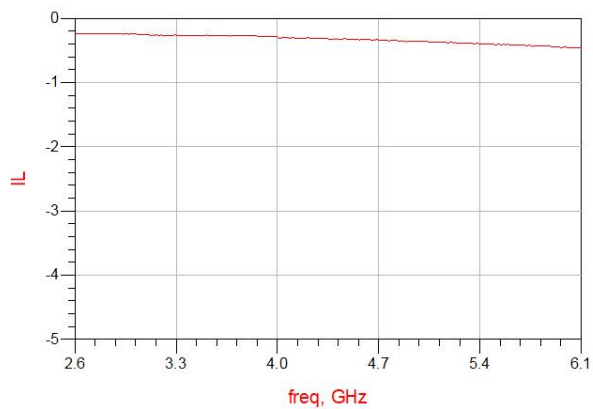
Figure 10. MHC4350E03 IL
