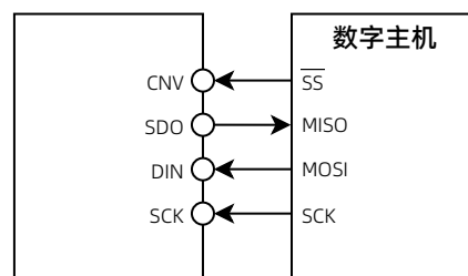
图 24 无繁忙指示器的连接图
