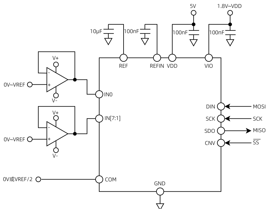
图 26 采用多个电源的应用电路
