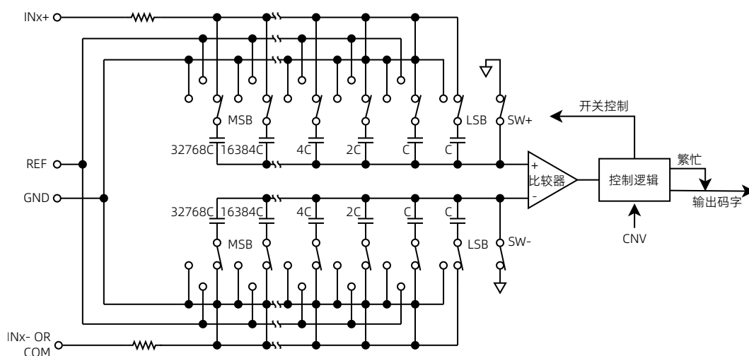
图 19 ADC 原理示意图
