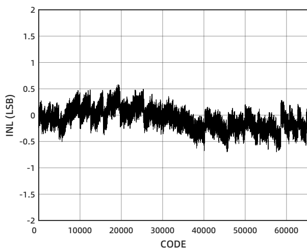
图 9 INL 误差
