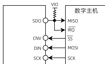
图 25 有繁忙指示器的连接图
