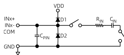
图 20 等效模拟输入电路
