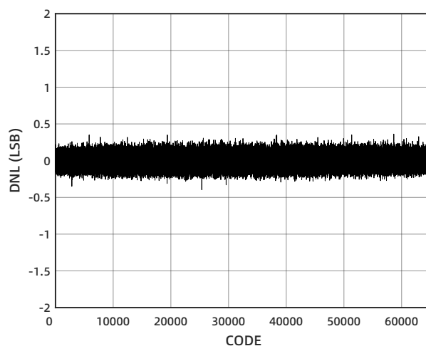
图 10 DNL 误差
