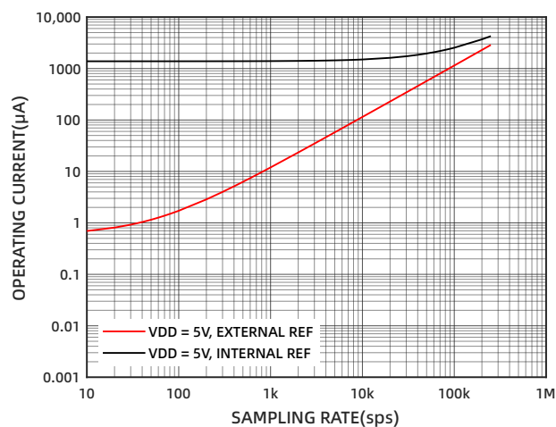
图 23 工作电流与采样率的关系
