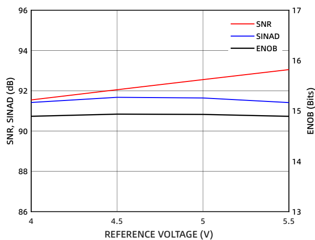
图 11 SNR、SINAD、ENOB 与基准电压的关系
