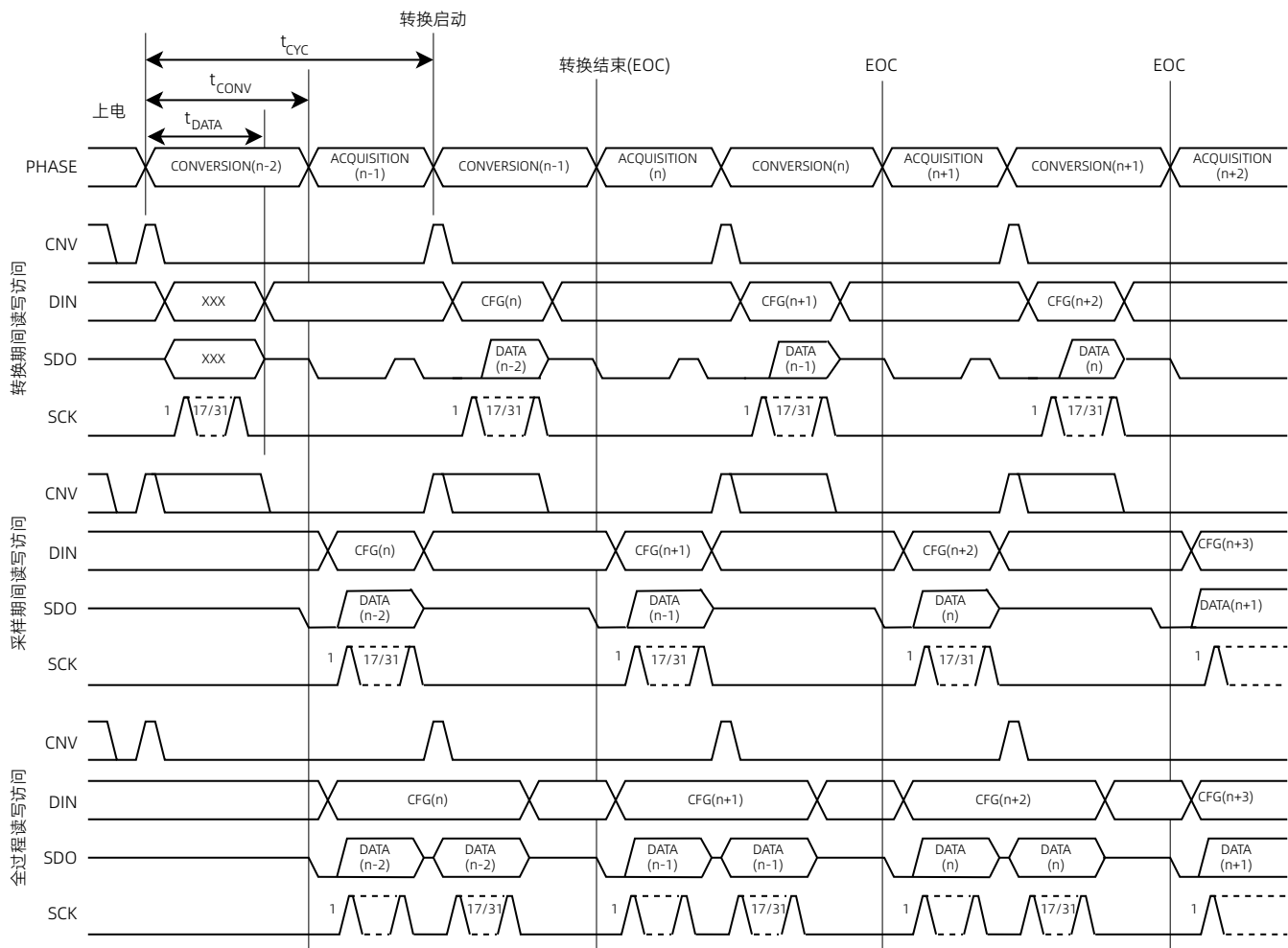
图 2 有繁忙指示器的通用接口时序
