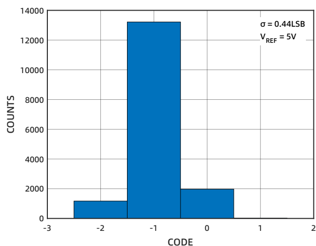
图 7 直流输入直方图（码中心，5V）
