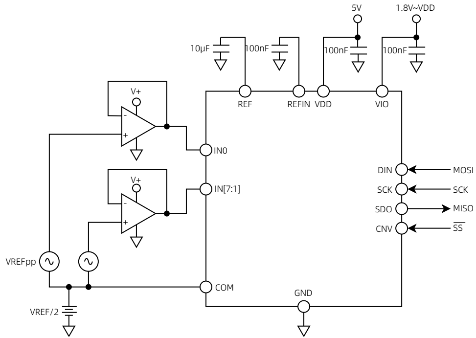
图 27 采用伪双极性输入的应用电路
