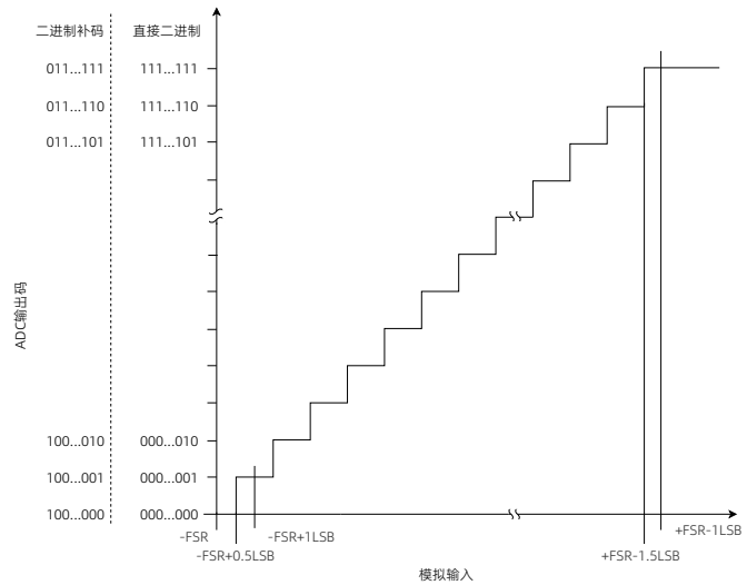
图 22 传递特性
