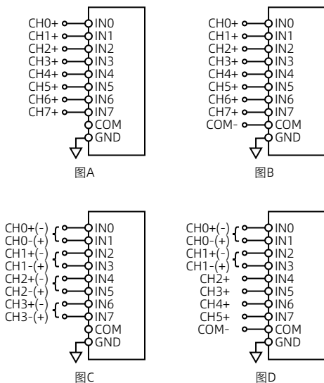
图 21 多路选择器模拟输入配置
