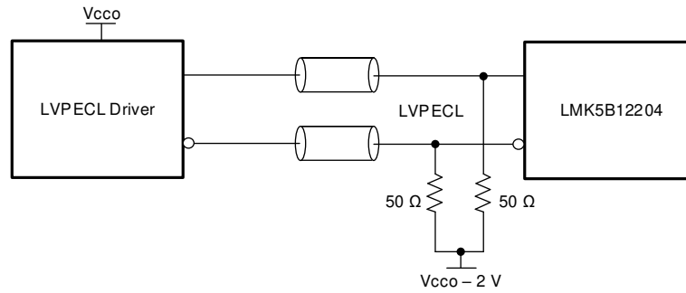
图 9-10. DC-Coupled LVPECL to Reference (PRIREF_P/SECREF_P) or XO Inputs
