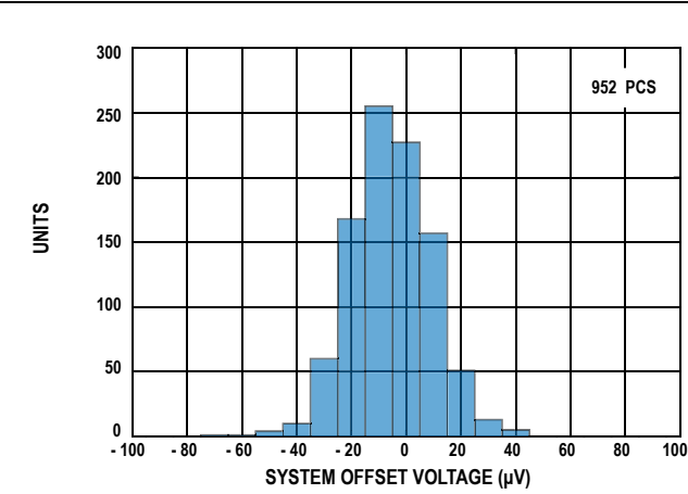
图6. 系统失调电压分布
