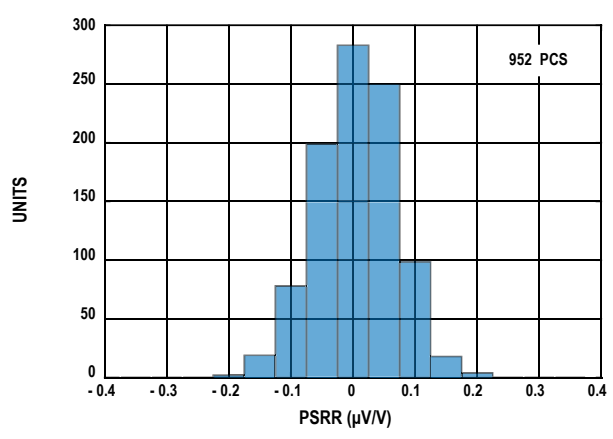
图12. PSRR 分布图
