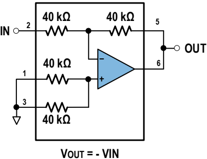
图42.增益为-1 的放大器
