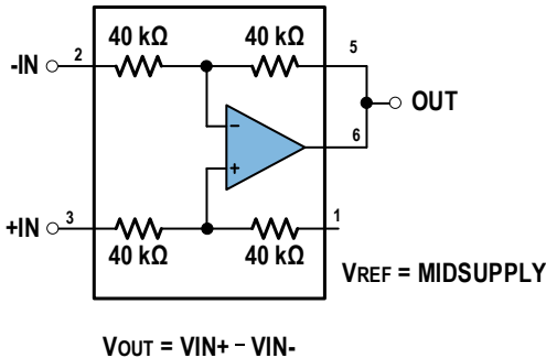
图41.差分放大器(增益为 1, V_{REF} 为供电电压的 1/2)
