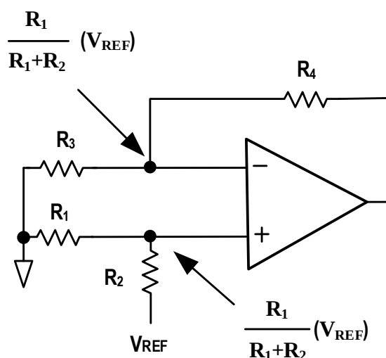
图38.确保内部运算放大器输入端有足够的电压摆动范围
