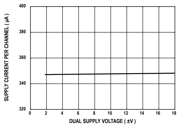
图25. 电源电流与双电源电压的关系( V_{IN} = 0\text{ V} )
