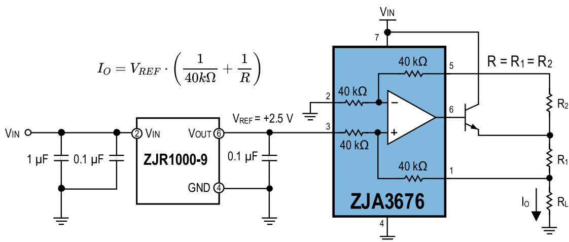
图47.用 ZJR1000 及 ZJA3676 实现精密恒流源
