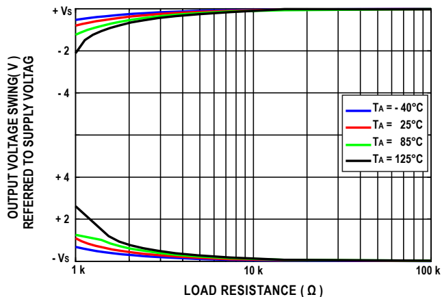
图21. 输出电压摆幅与负载电阻的关系 ( V_s = \pm 15\text{ V} )
