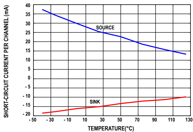
图23. 短路电流与温度的关系
