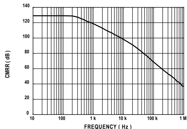
图15. CMRR 与频率的关系
