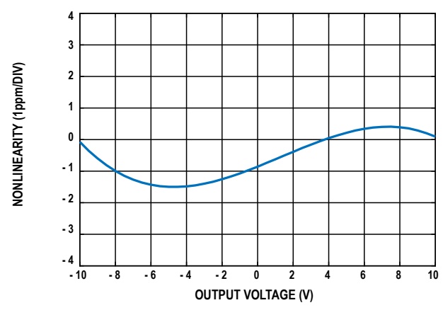
图28. 增益非线性度( V_S = \pm 15\text{ V} , R_L \geq 2\text{ k}\Omega )
