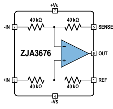
图2. ZJA3676 功能框图
