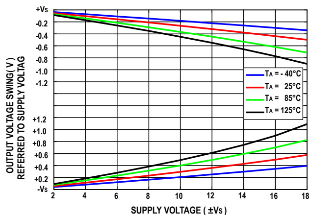
图19. 输出电压摆幅与电源电压的关系 ( R_L = 2\text{ k}\Omega )
