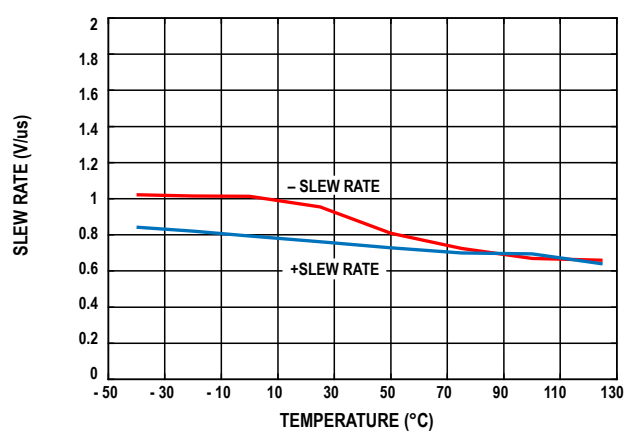
图24. 压摆率与温度的关系( V_{IN} = 20\text{ V}_{P-P} , 1 kHz)
