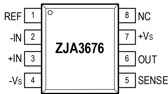
图3. ZJA3676 管脚排列图 (SOIC-8 封装)
