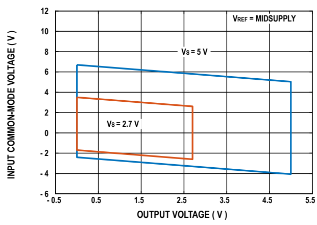
图17. 输入共模电压与输出电压的关系 (单电源供电, V_{REF} = \text{MIDSUPPLY} )
