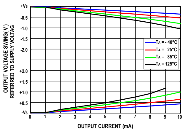
图22. 输出电压摆幅与输出电流的关系 ( V_s = \pm 15\text{ V} )
