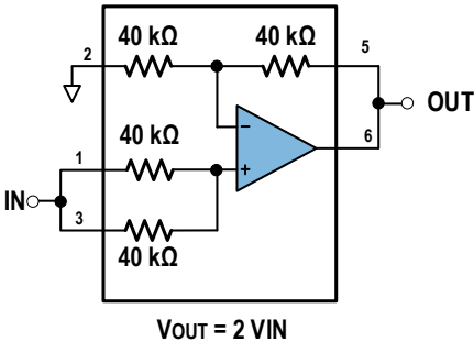
图44.增益为 2 的放大器
