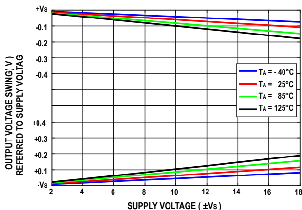
图20. 输出电压摆幅与电源电压的关系 ( R_L = 10\text{ k}\Omega )
