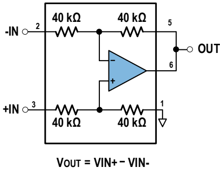
图40.差动放大器(增益为 1)
