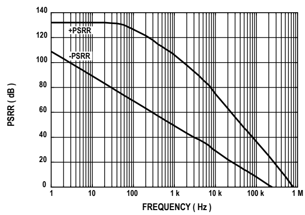
图13. PSRR 与频率的关系
