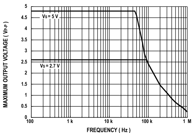
图30. 最大输出电压与频率的关系( V_s = 5\text{ V}, 2.7\text{ V} )
