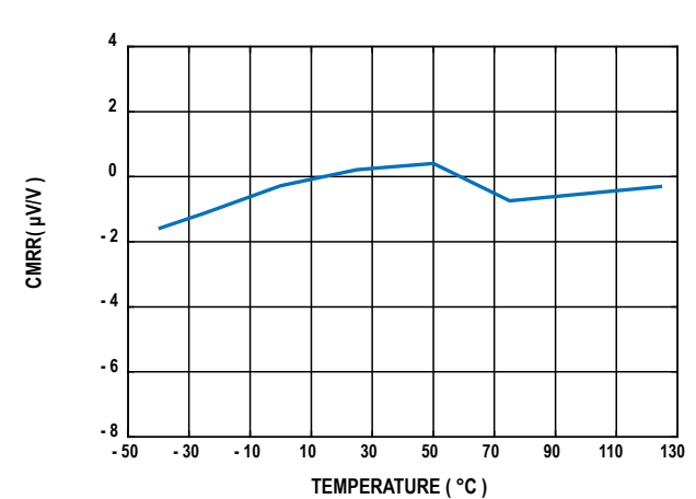
图9. 共模抑制比 CMRR 与温度的关系
