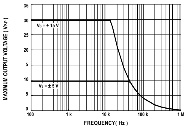
图29. 最大输出电压与频率的关系( V_S = \pm 15\text{ V} , \pm 5\text{ V} )
