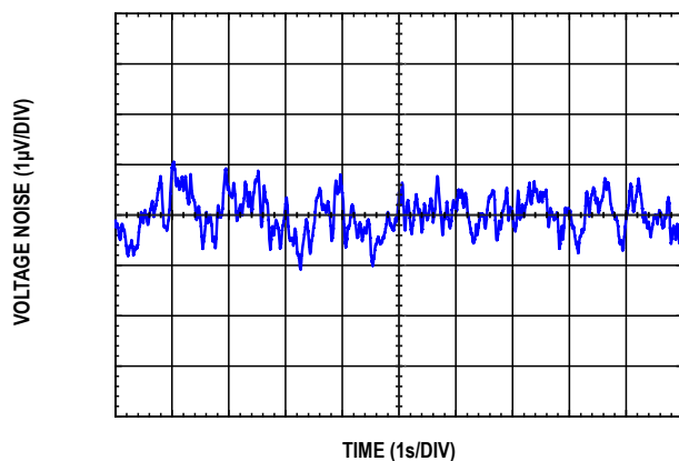
图35. 0.1 Hz 至 10 Hz 噪声
