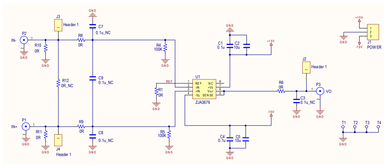
图51.ZJA3676 评估板原理图
