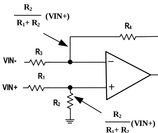
图37.差动放大器内部的电压情况
