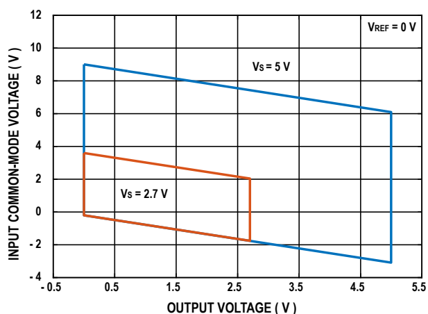
图18. 输入共模电压范围与输出电压的关系 (单电源供电, V_{REF} = 0\text{ V} )
