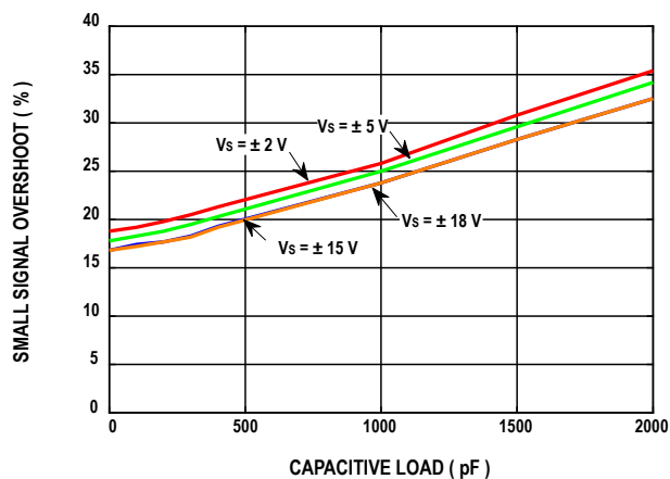
图33. 小信号过冲与负载电容的关系( R_L \geq 2\text{ k}\Omega )
