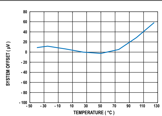
图7. 系统失调电压与温度的关系
