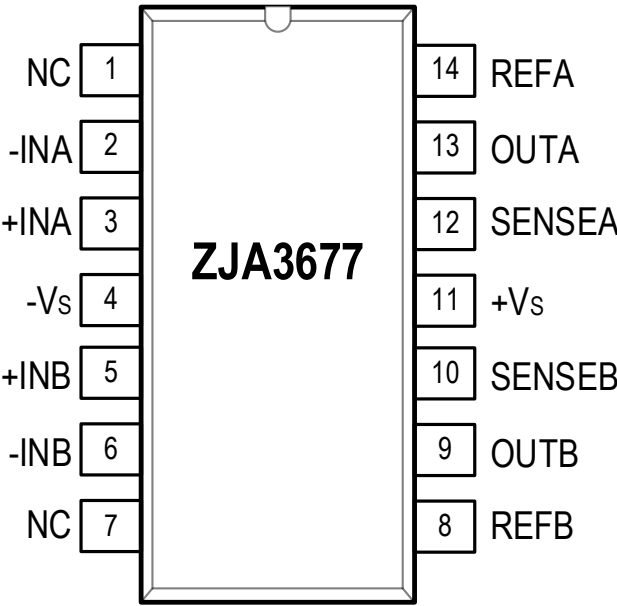
图5. ZJA3677 管脚排列图 (SOIC-14 封装)
