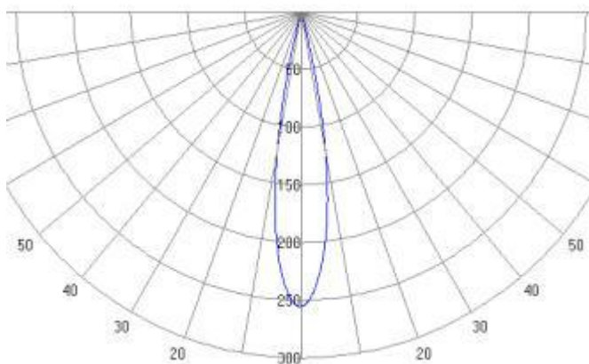
配光曲线-极坐标
