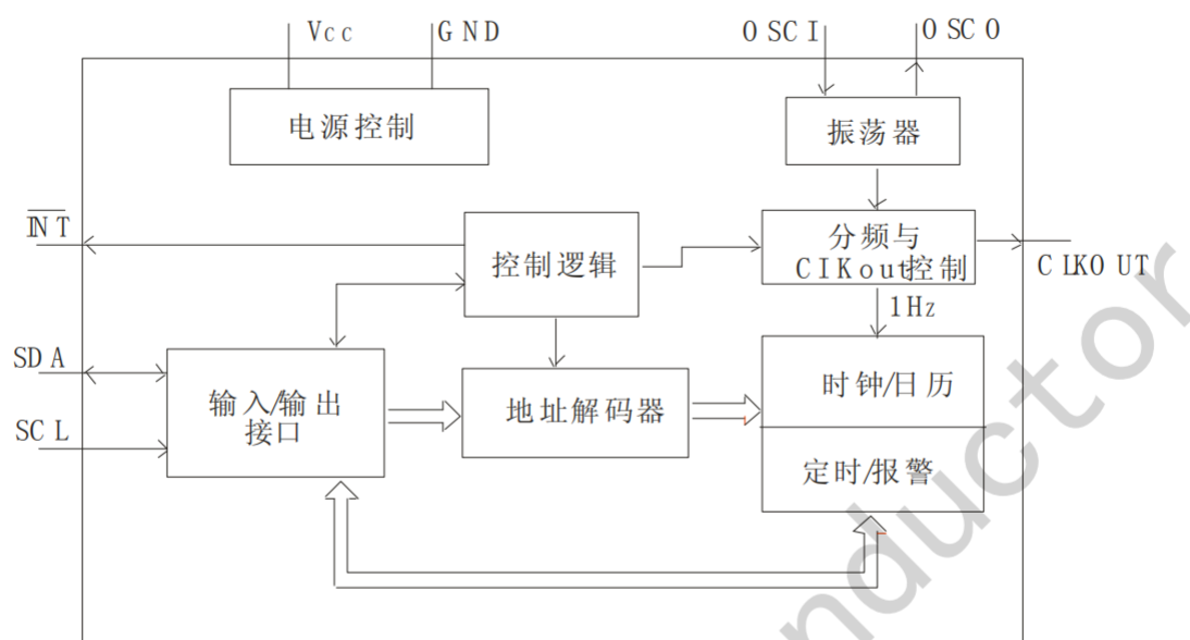
图 2. 方框图
