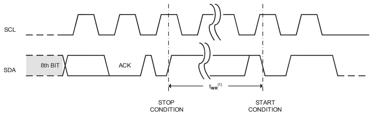
图2 总线时序
