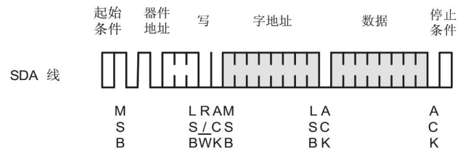
图9 字节写
