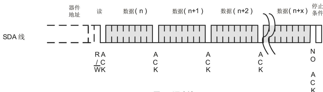
图14 顺序读
