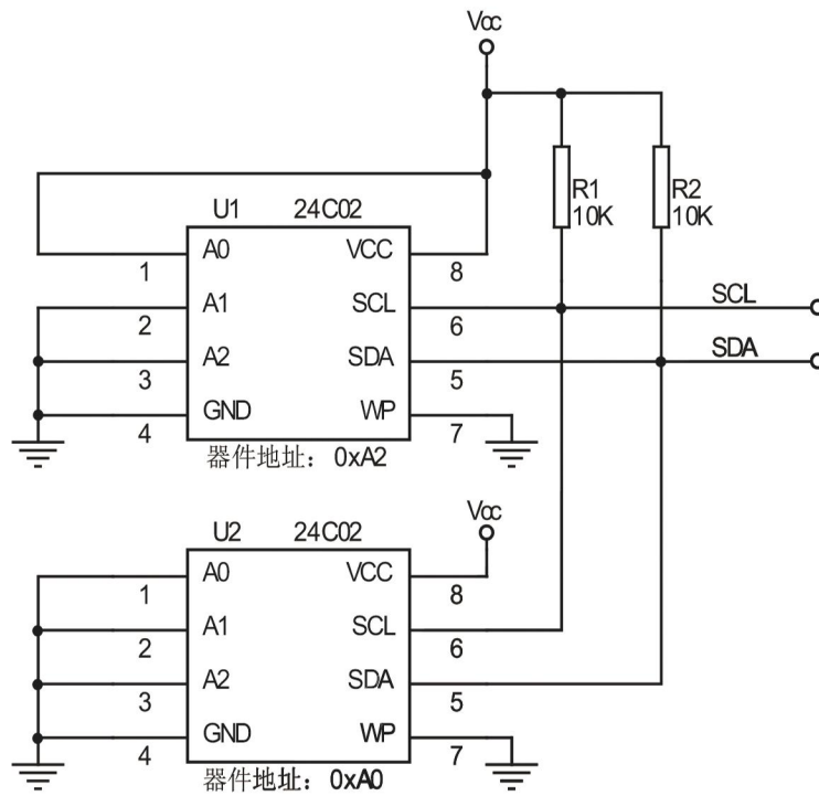
图15 EEPROM的级联
