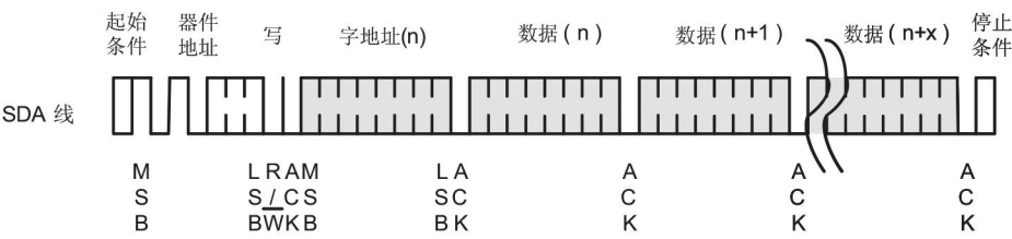
图10页写
