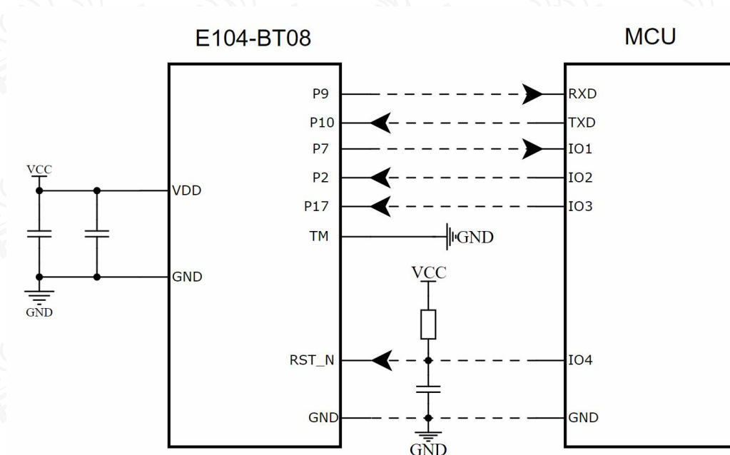
Figure 4-2 E104-BT08 Circuit
